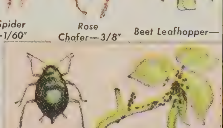
Bean Aphid—3/32"
