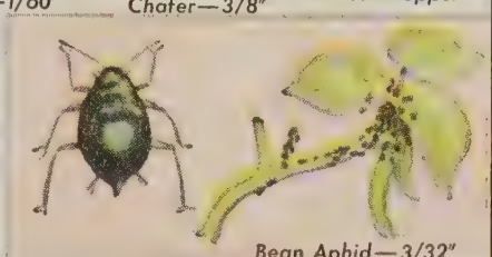
Bean Aphid—3/32"
