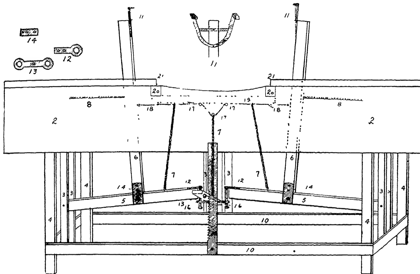
Fig 22. Clamp Nailing Press
