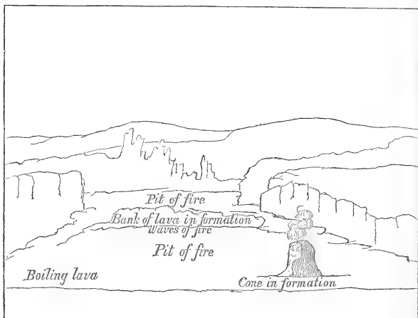
Halemaumau, Jan. 31.
