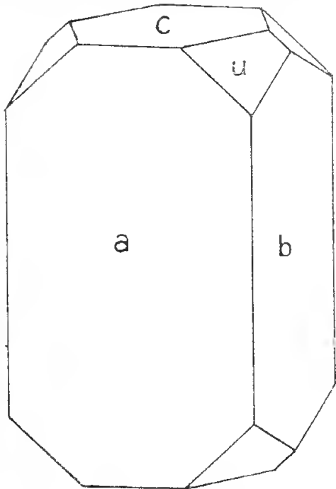
Fig. 19. Manganocolumbite, Tappa.
