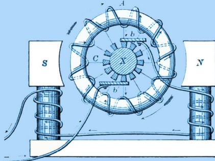
FIG. 40.—A Dynamo.
