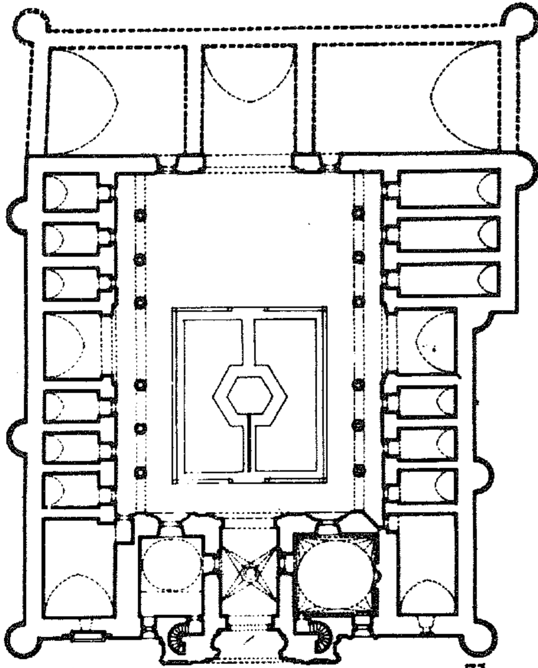
مسقط أفقى لمدرسة جوك بسيفاس
