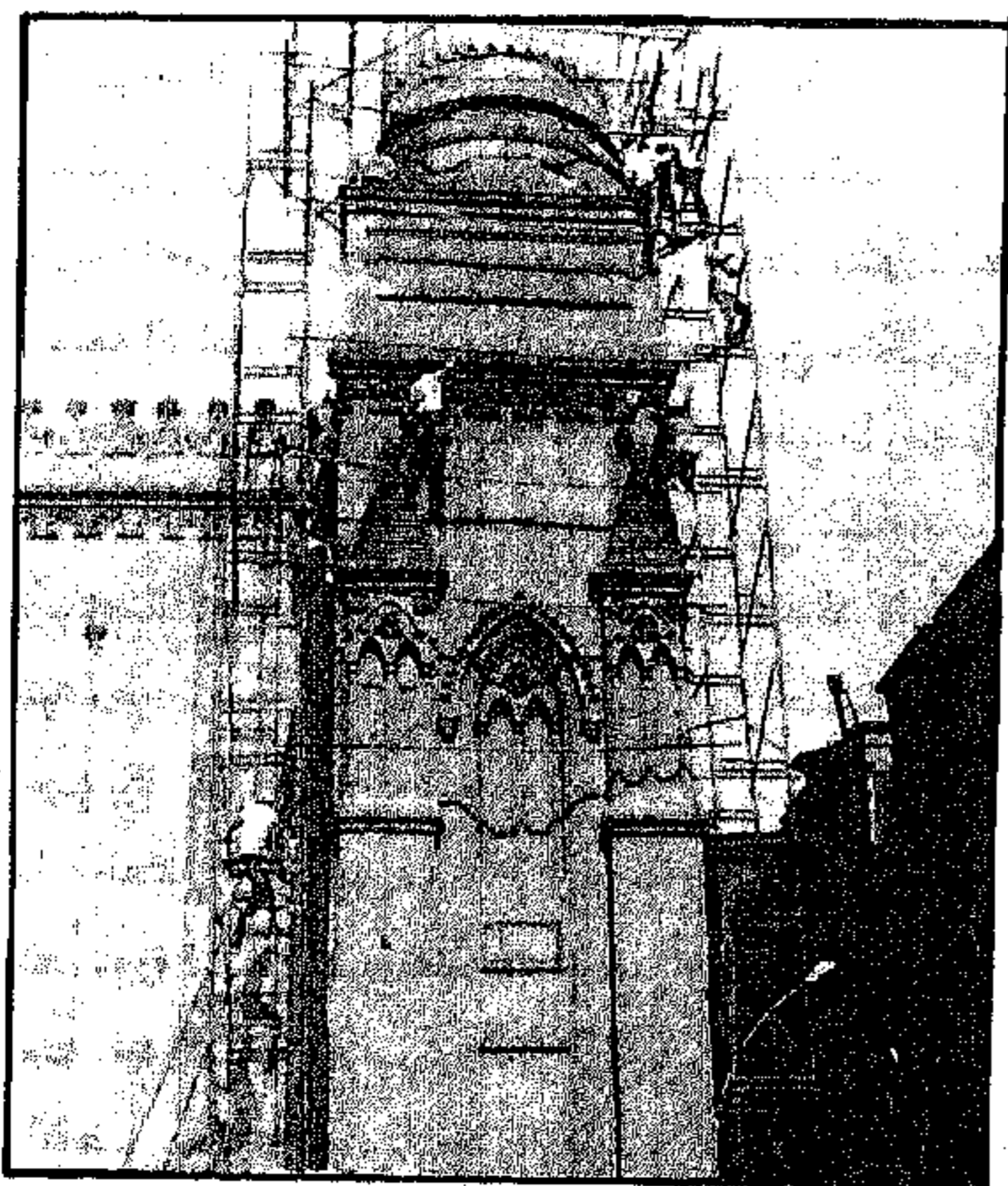
أعمال التنظيف الميكانيكي للمنارة الغربية .
