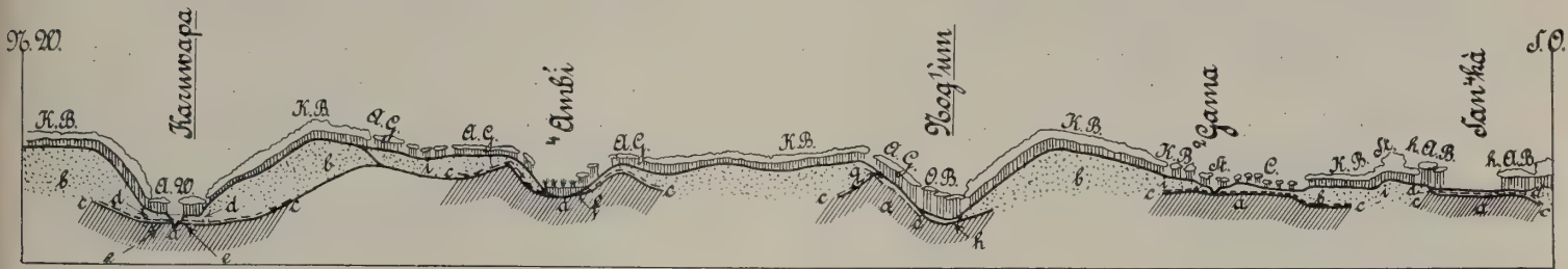
Schemat. Profil des Omatako-Tales am nördl. Gorósumpf.
