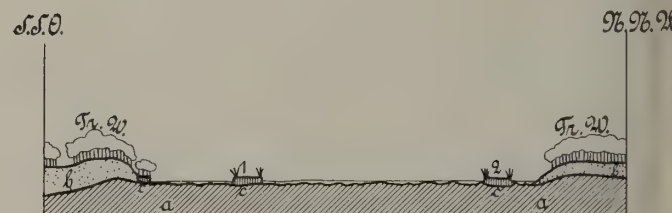
Schematisches Profil durch das Okavangotal am oberen Rande der Popafälle.
