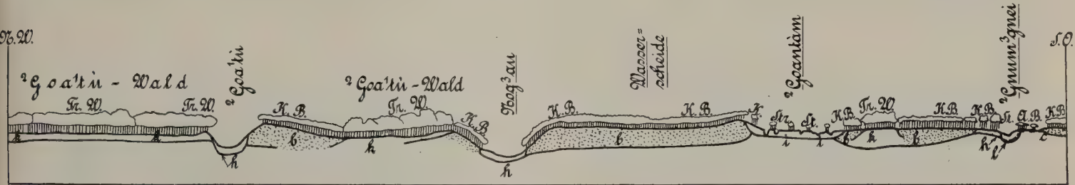
Schematisches Profil durch das nördliche Sandfeld von Karuwapa bis Sankhá.
