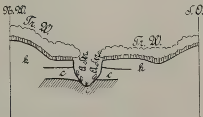
Schemat. Profil durch die Talenge des Omatako an den Löwenfüßen. Sehr stark überhöht.
