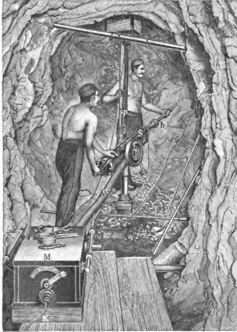
Elektrisch angetriebene Stoßbohrmaschine v. Siemens & Halske.
