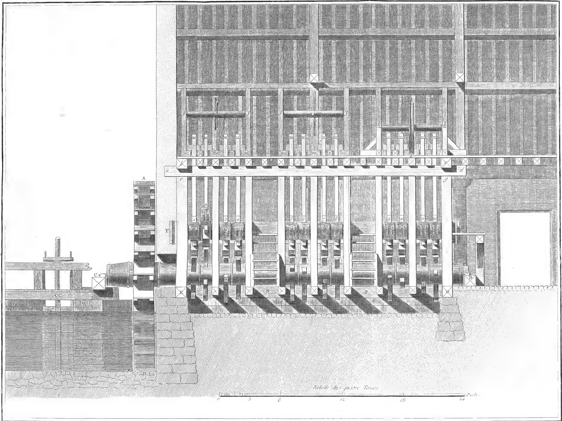
Tanneur, Élévation du Moulin pour les Buffles.
