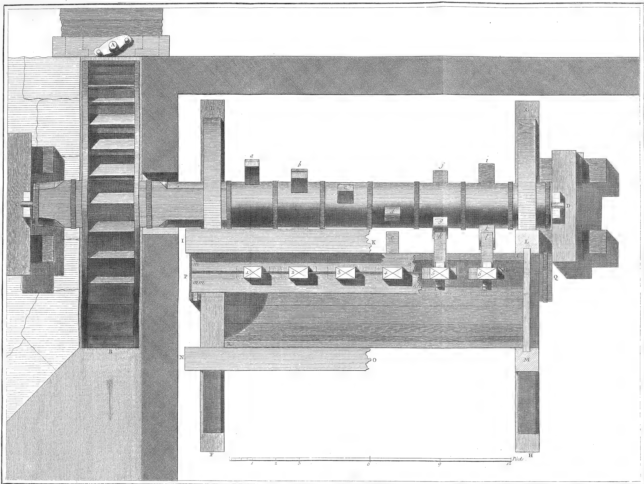
Tanneur, Plan Général du Moulin à Tan.
