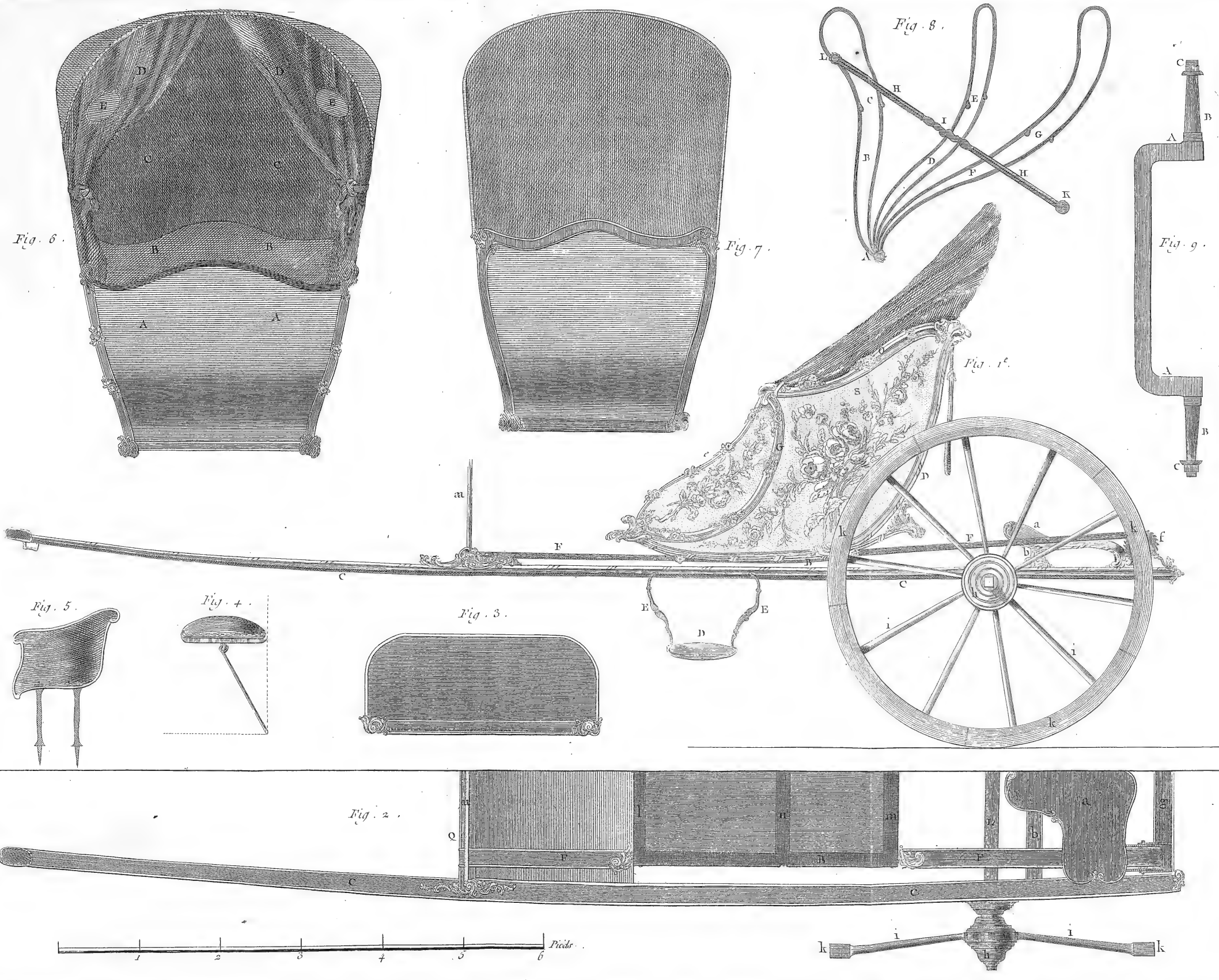
Sellier - Carrossier, chaise ou cabriolet.
