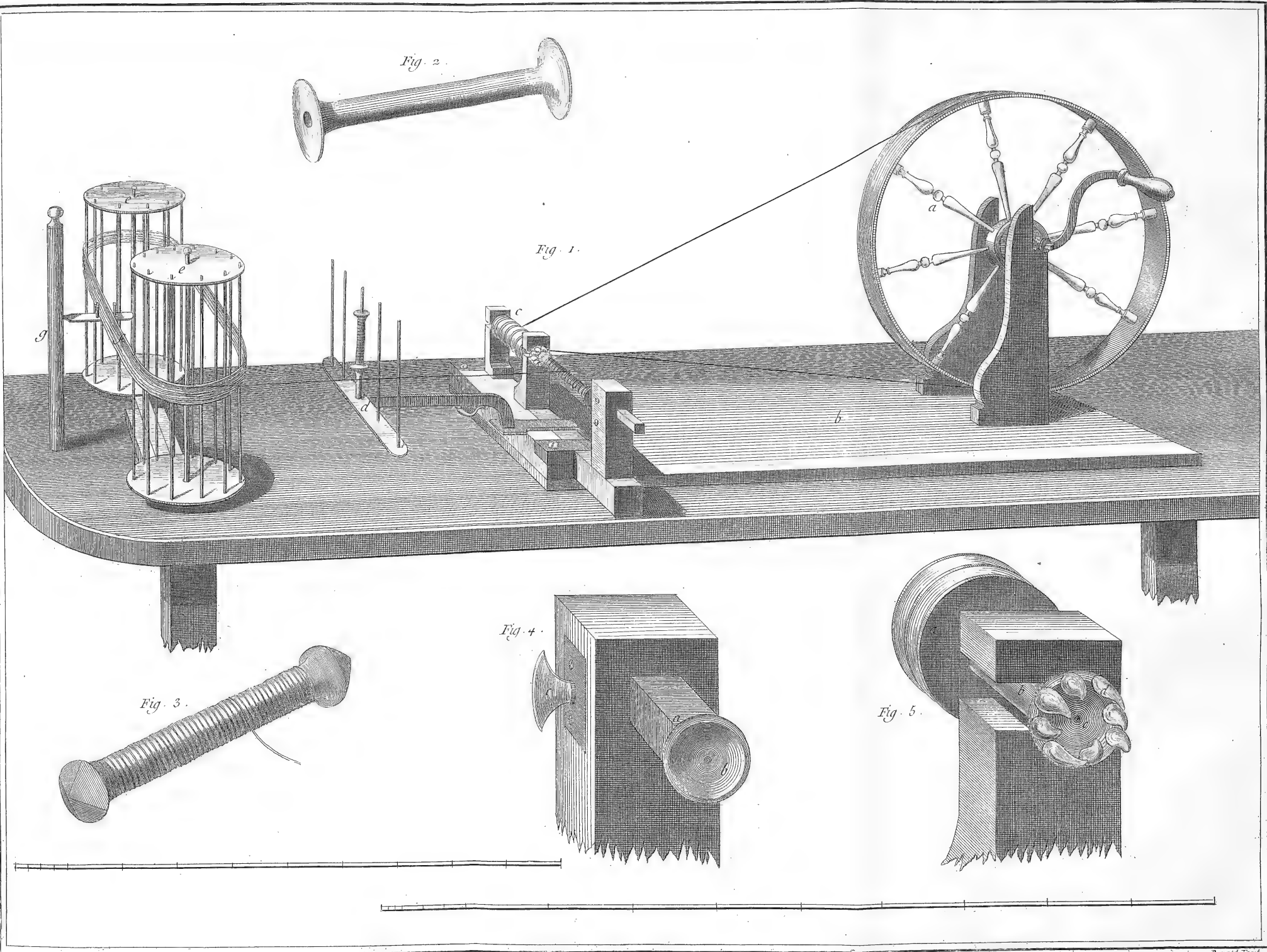
Tapisserie de Basse Tisse des Gobelins, Rouet à devider les laines sur les Bobines et sur les Flattes, et Développemens.
