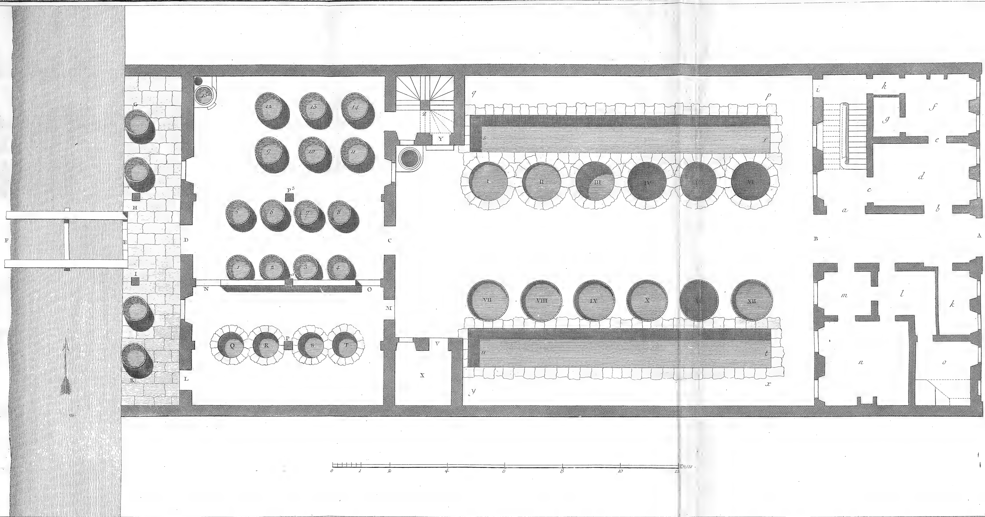
Tanneur, Plan Général d'une Tannerie.
