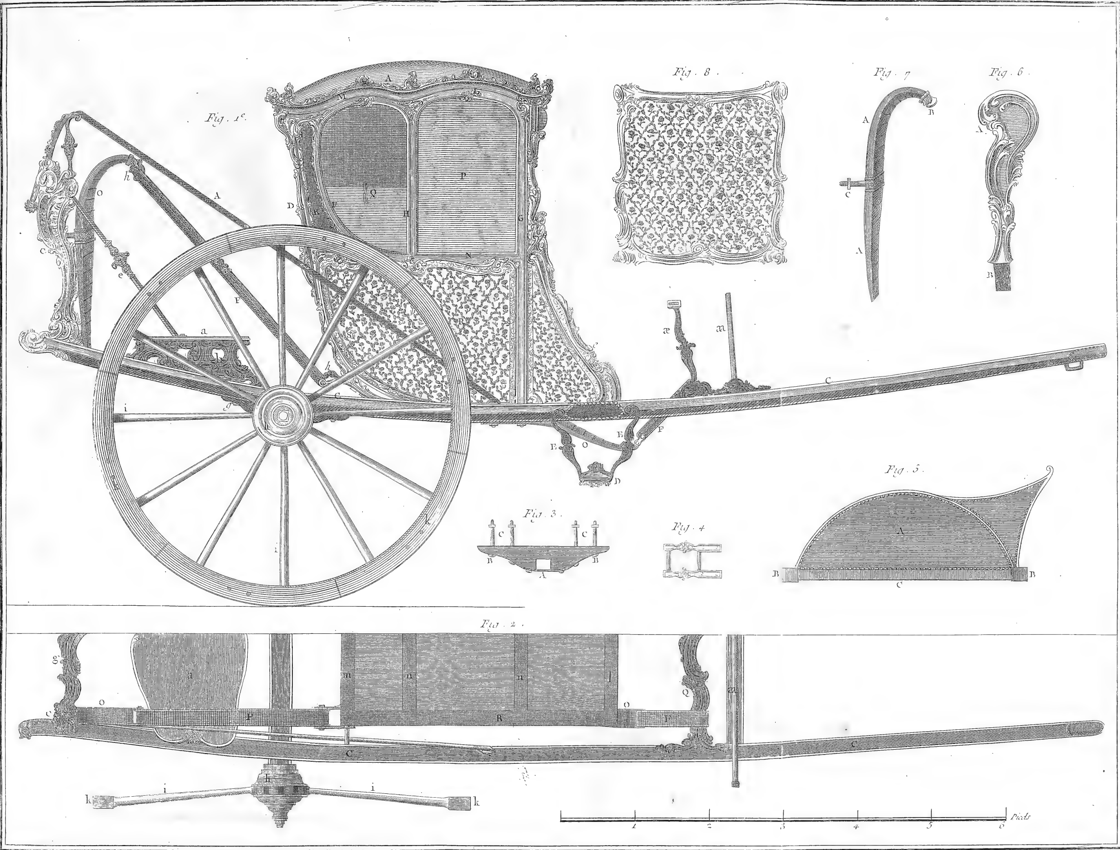
Sellier-Carrossier, chaise de Poste à cul de Singe.
