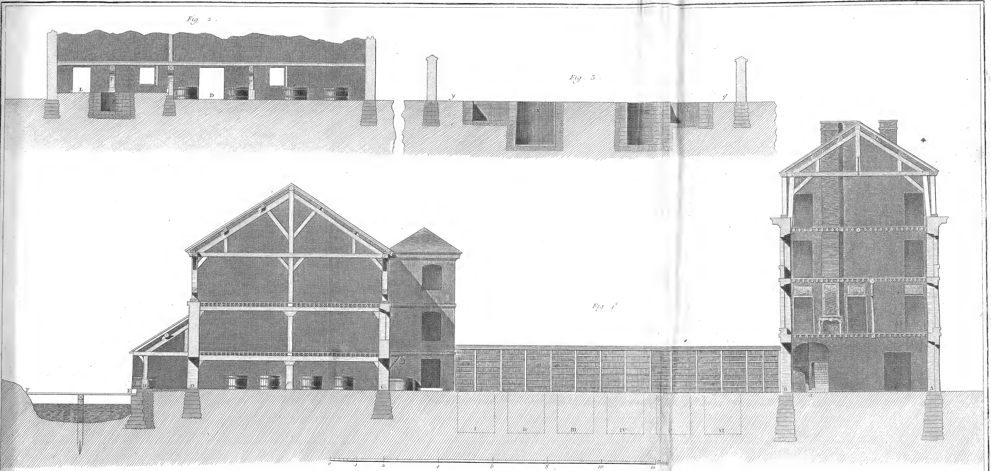
Tanneur, Coupes Longitudinale et Transversalle de la Tannerie.
