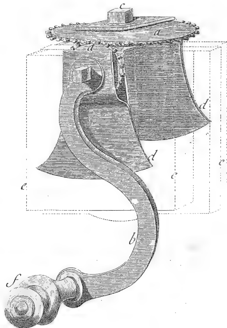
Tapissierie de Haute Lisse des Gobelins , Vue du Mélétier monté avec la nouvelle machine pour faciliter le bandage des fils et avec deux Hommes seulement ; Développement de cette Machine
