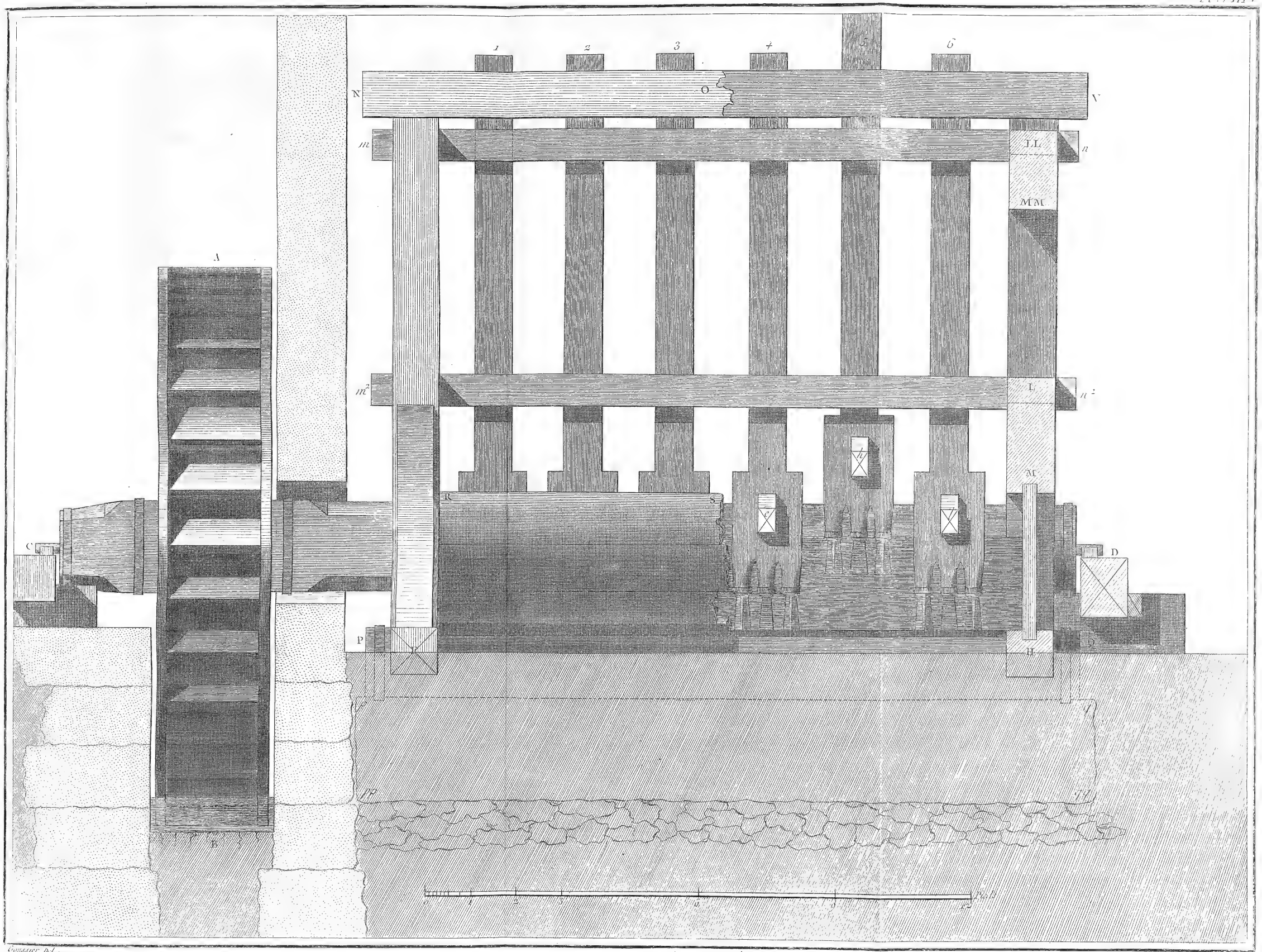
Tanneur, Élévation Antérieure du Moulin à Tan.
