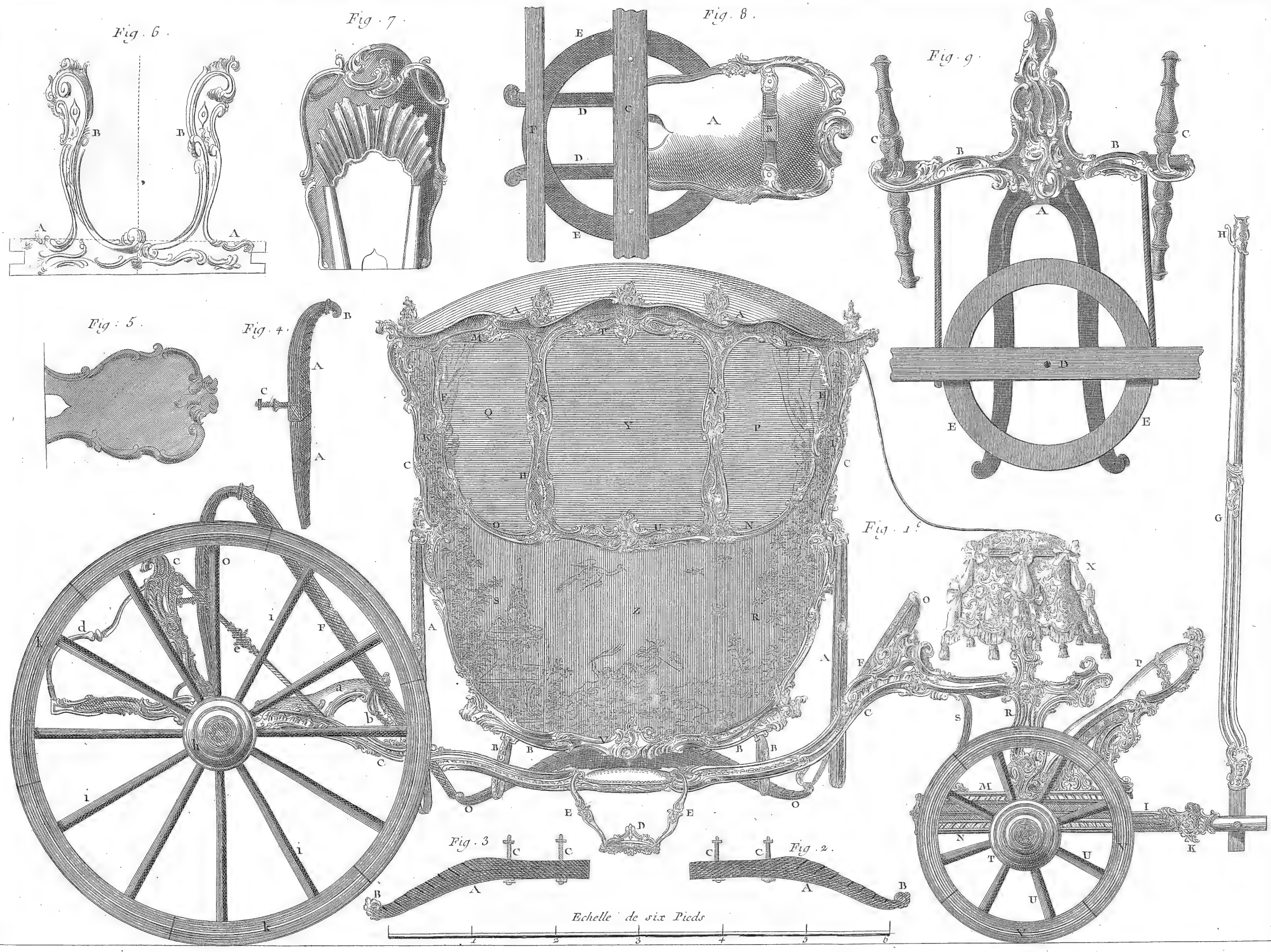
Sellier-Carrossier, Berlin ou vis-à-vis à panneaux arrasés.
