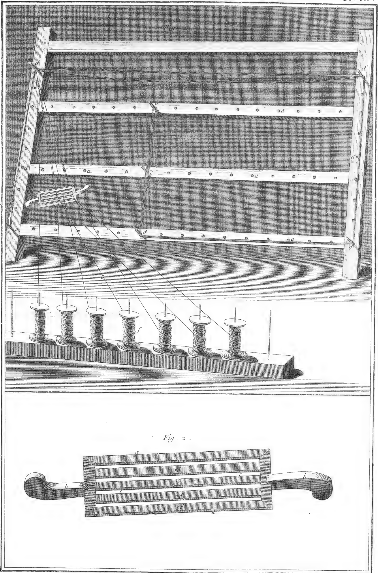
Tapisserie de Basse-Lisse des Gobelins, Proportions et Service de l'Ourdissoir, et Outils pour les fils de croisure de l'Ourdisage.
