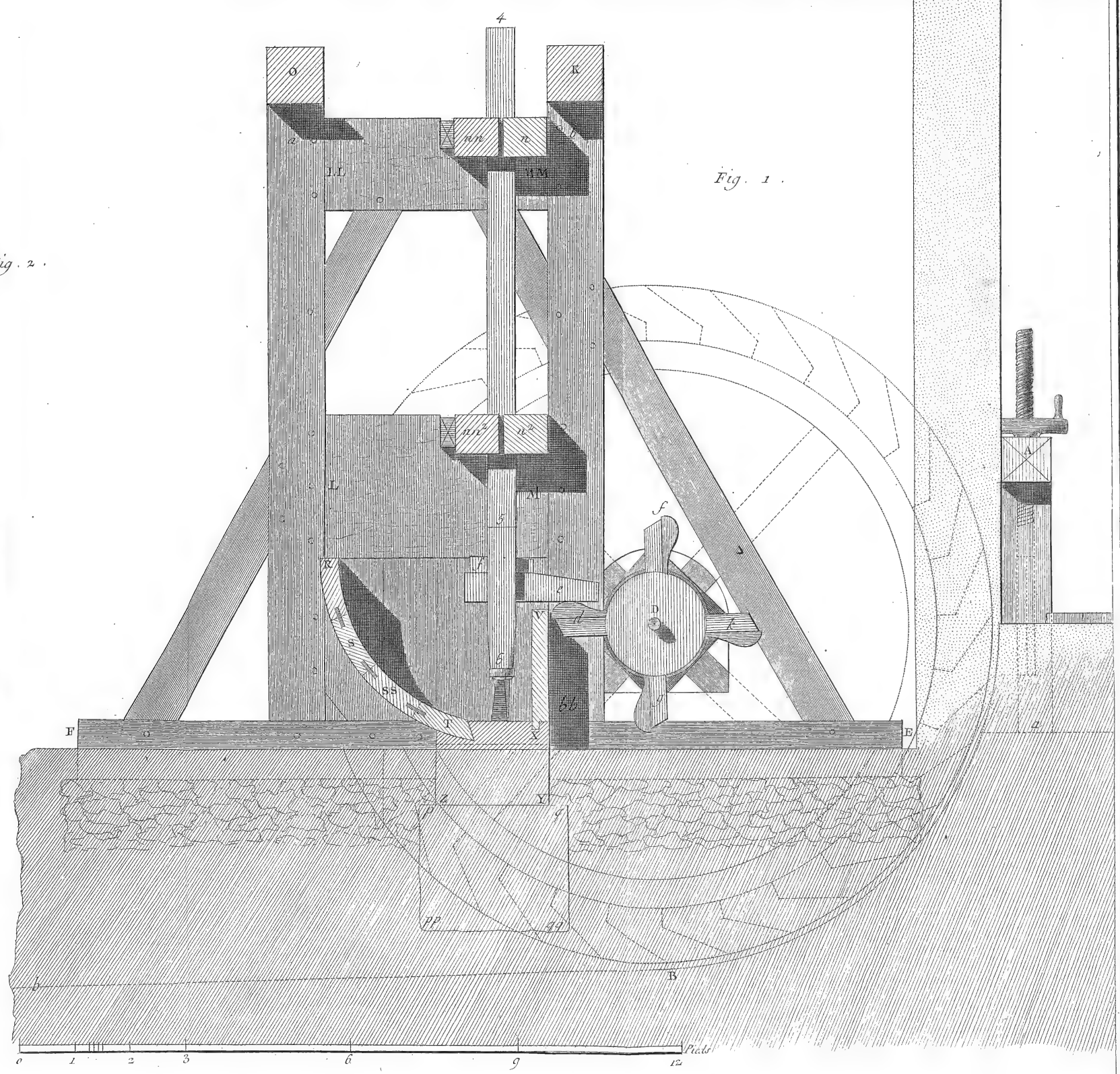
Tanneur, Coupe Transversalle du Moulin à Tan.
