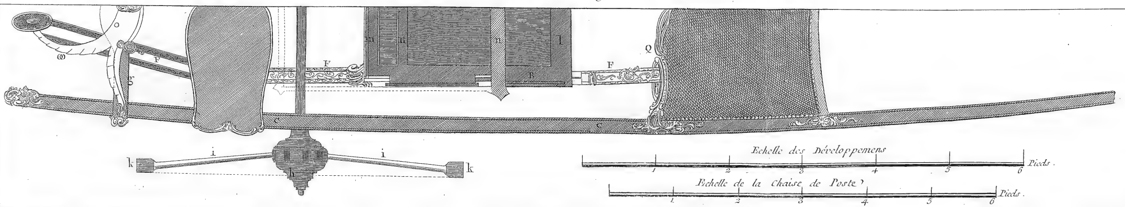
Sellier-Carrossier, chaise de Poste à l'Écrivoise.
