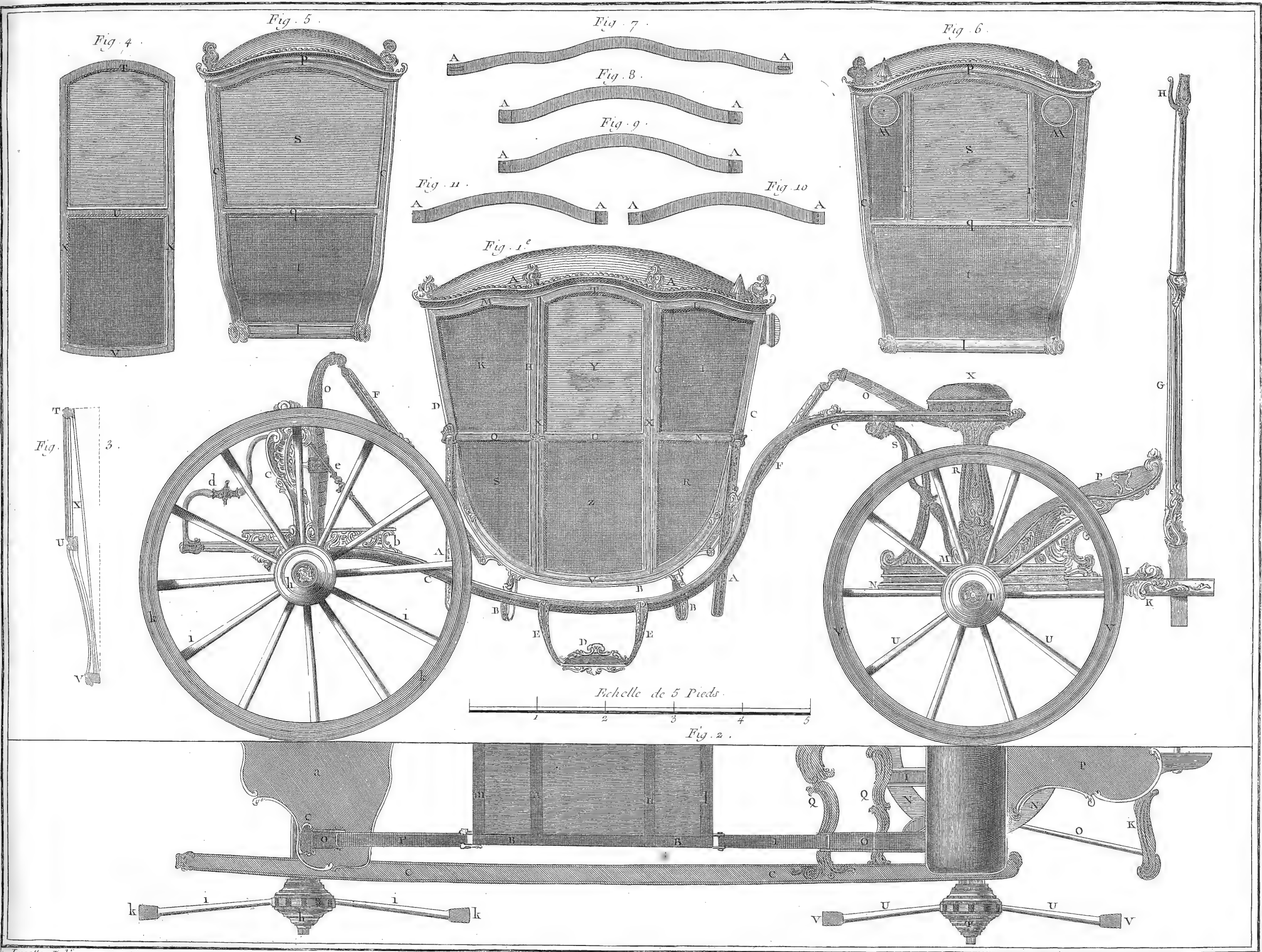
Sellier-Carrossier, Berline de Campagne à Cul de Singe.
