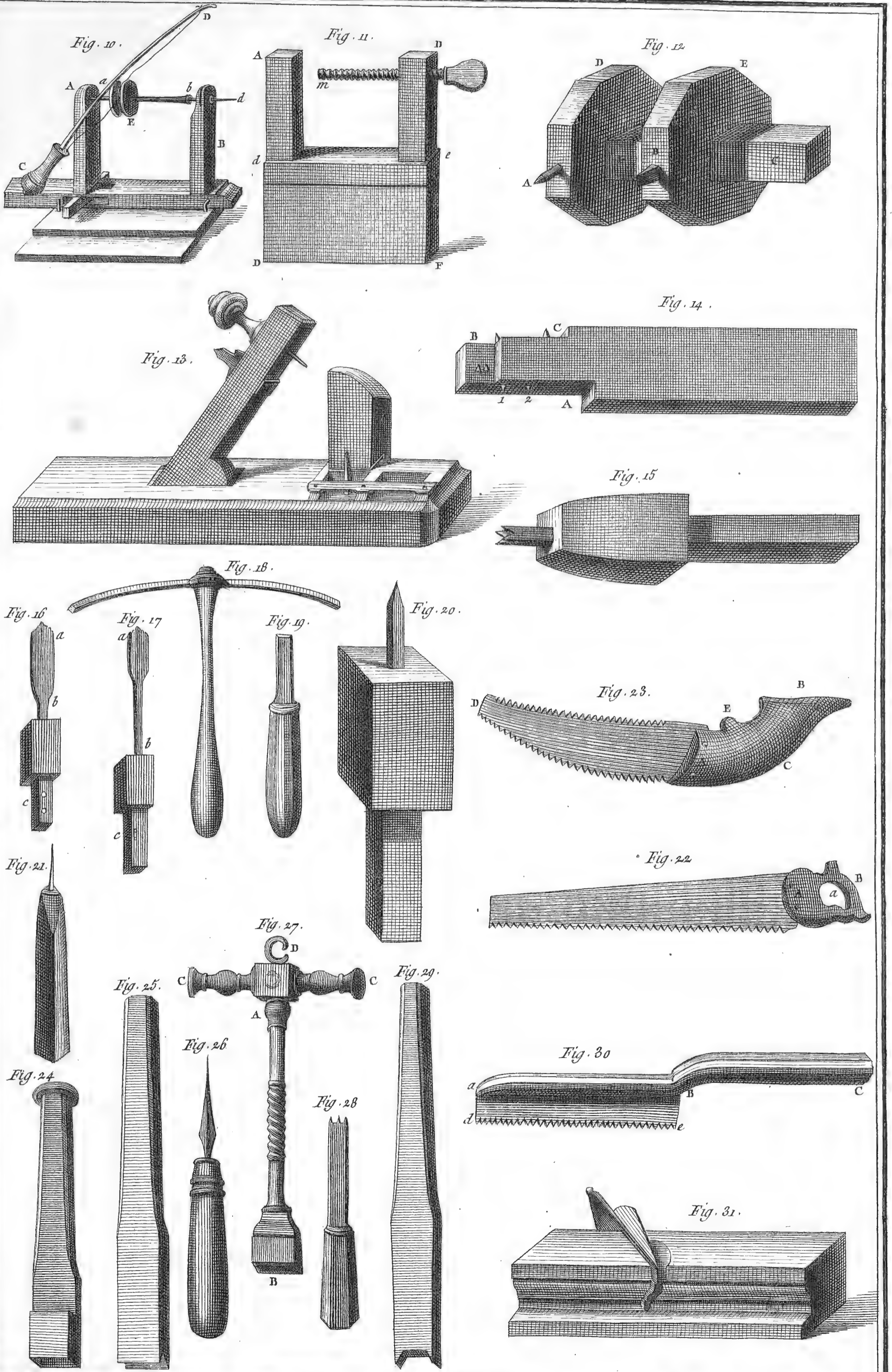
Lutherie, outils propres à la Façture des Clavecins.
