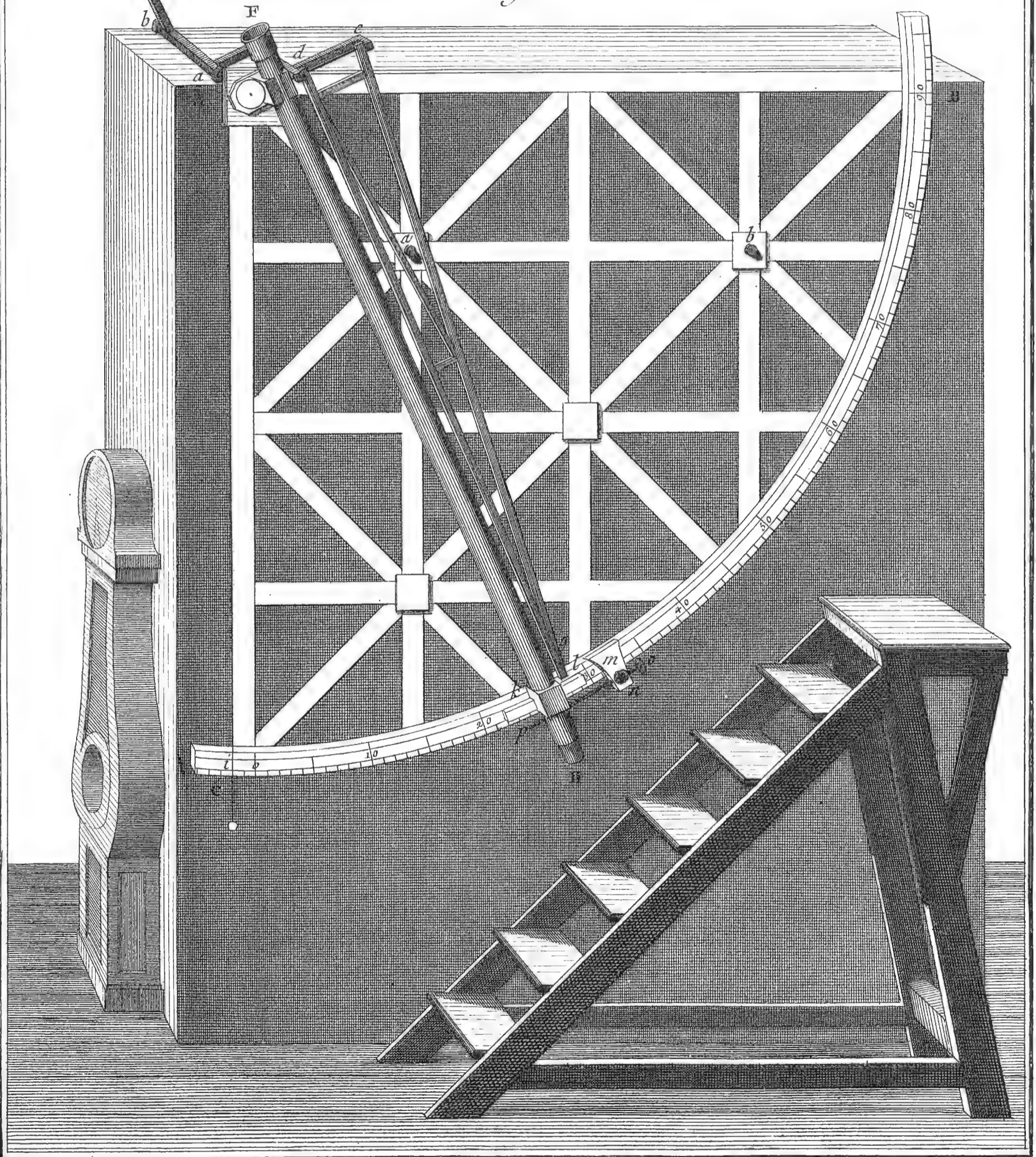
Astronomie Instrumens, Quart de cercle Mural en Perspective et Développement du Contrepoid de la Lunette.
