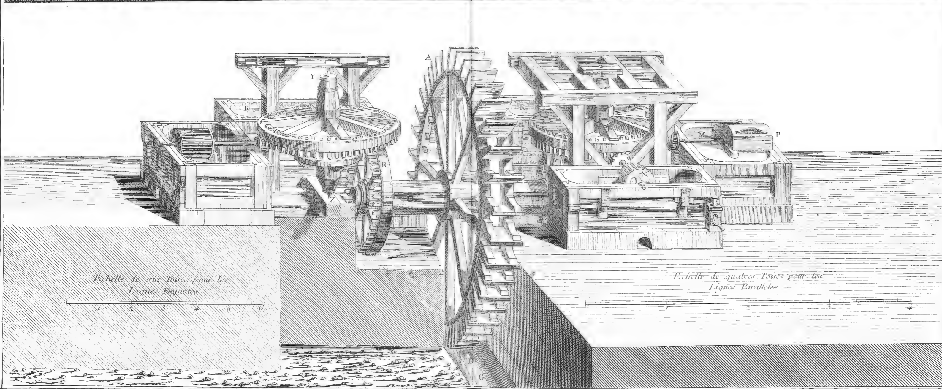
Papetterie, Vue des Bâtimens de la Manufacture de l'Anglée, près Montargis. Vue du Rouage d'un des Moulins de cette Manufacture.
