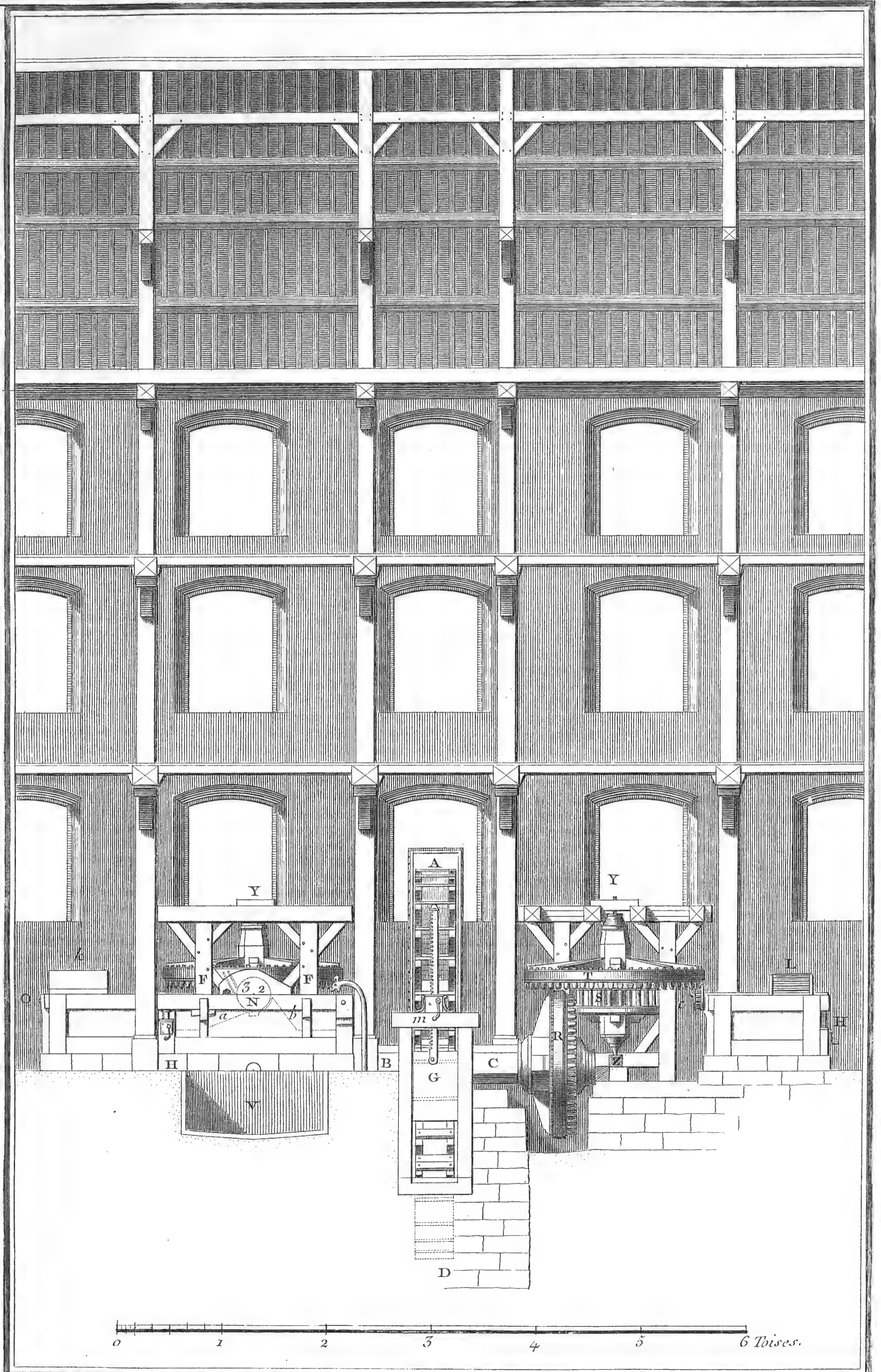
Papetterie, Moulin en Élévation.
