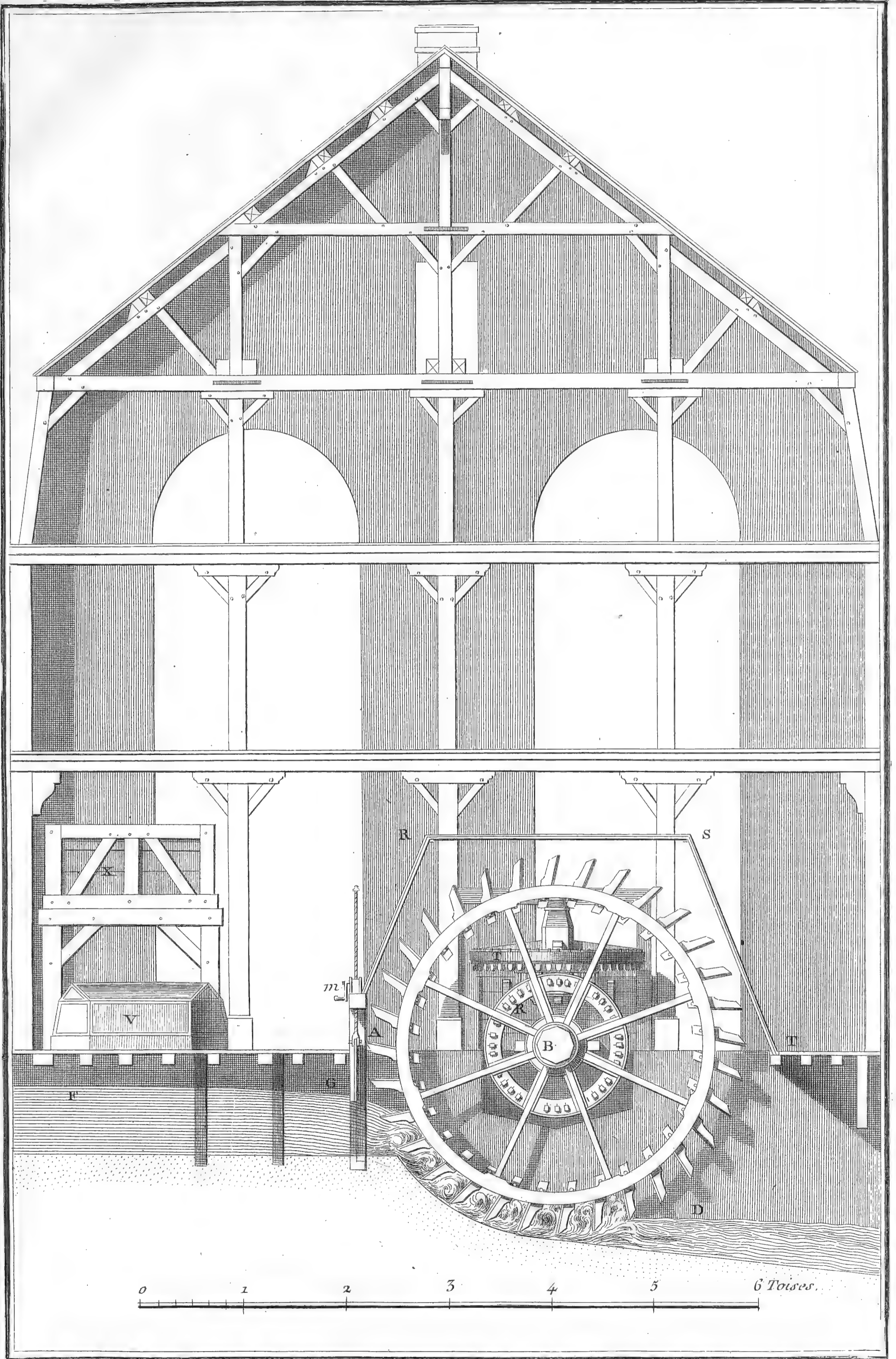
Papetterie, Moulin en Profil.
