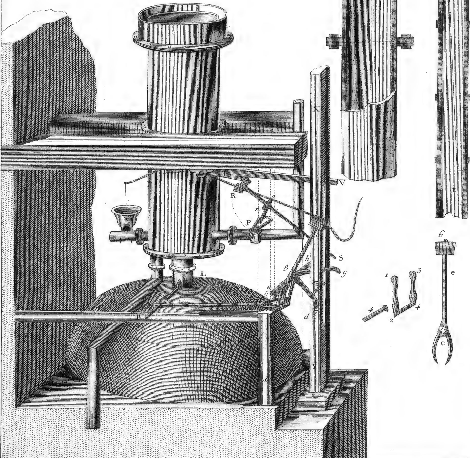
Hidraulique, Pompe a Feu Coupes et profils du Cilindre.
