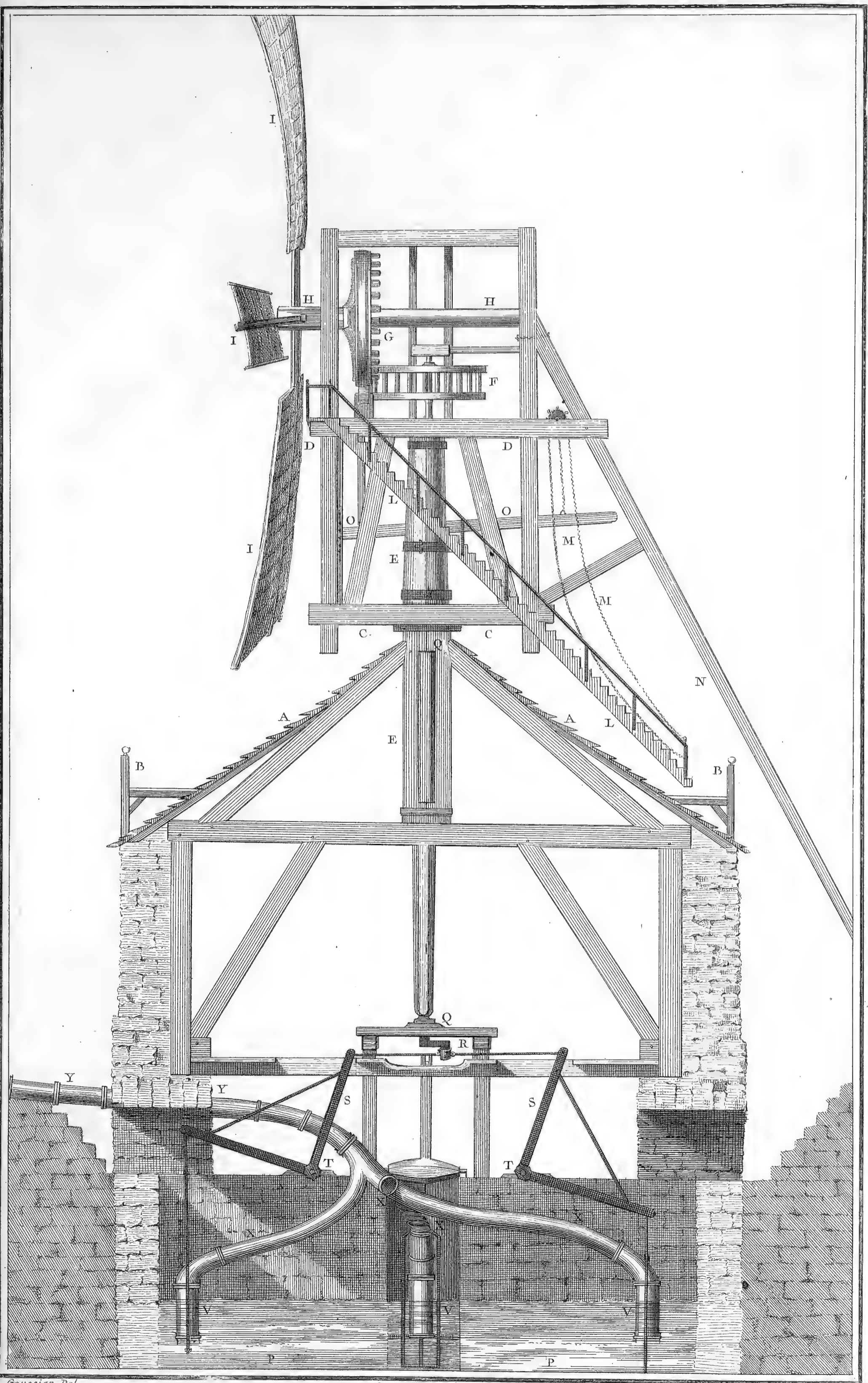
Hydraulique, Moulin à vent de Meudon.
