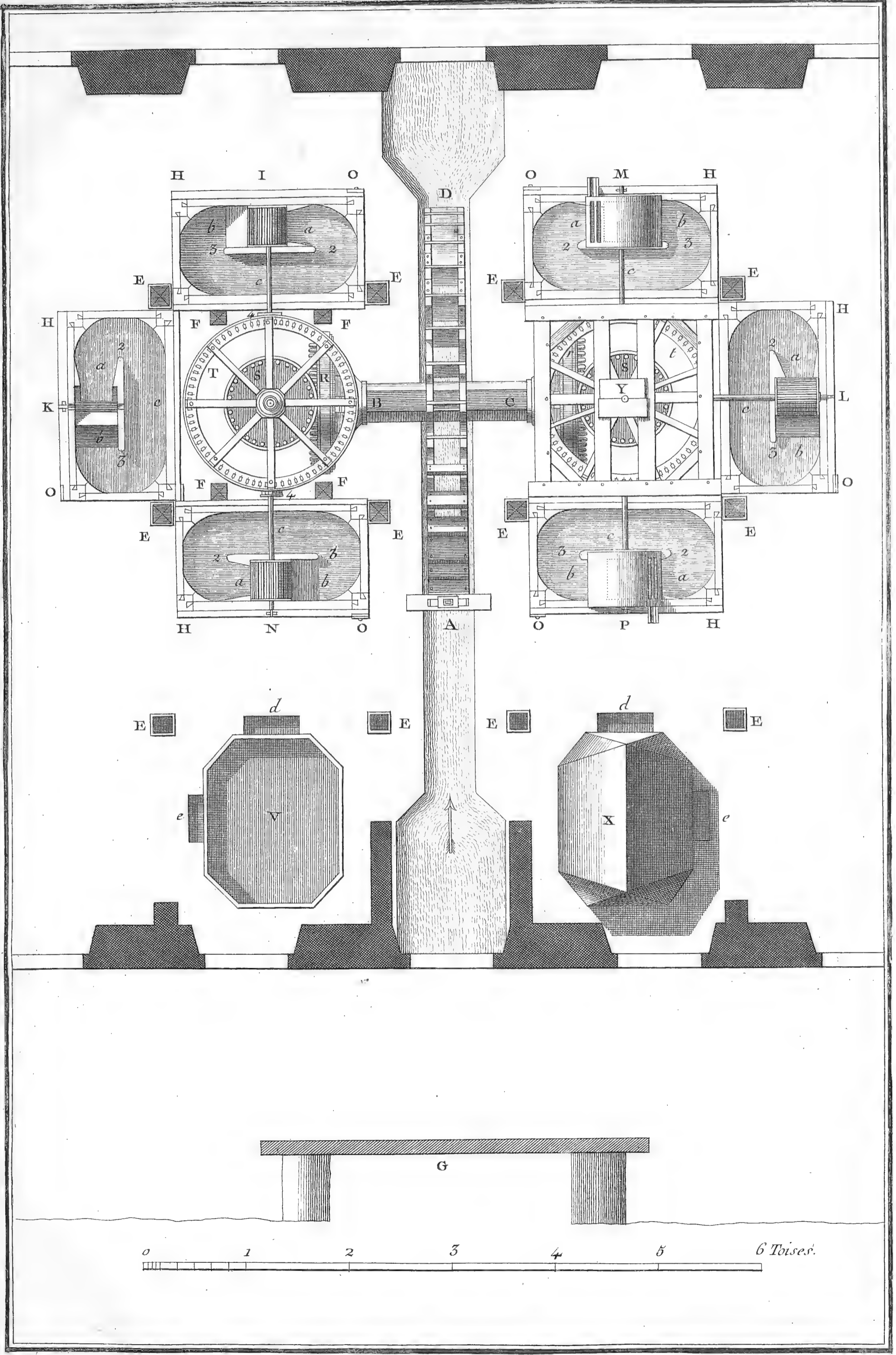
Papetterie, Moulin en Plan.
