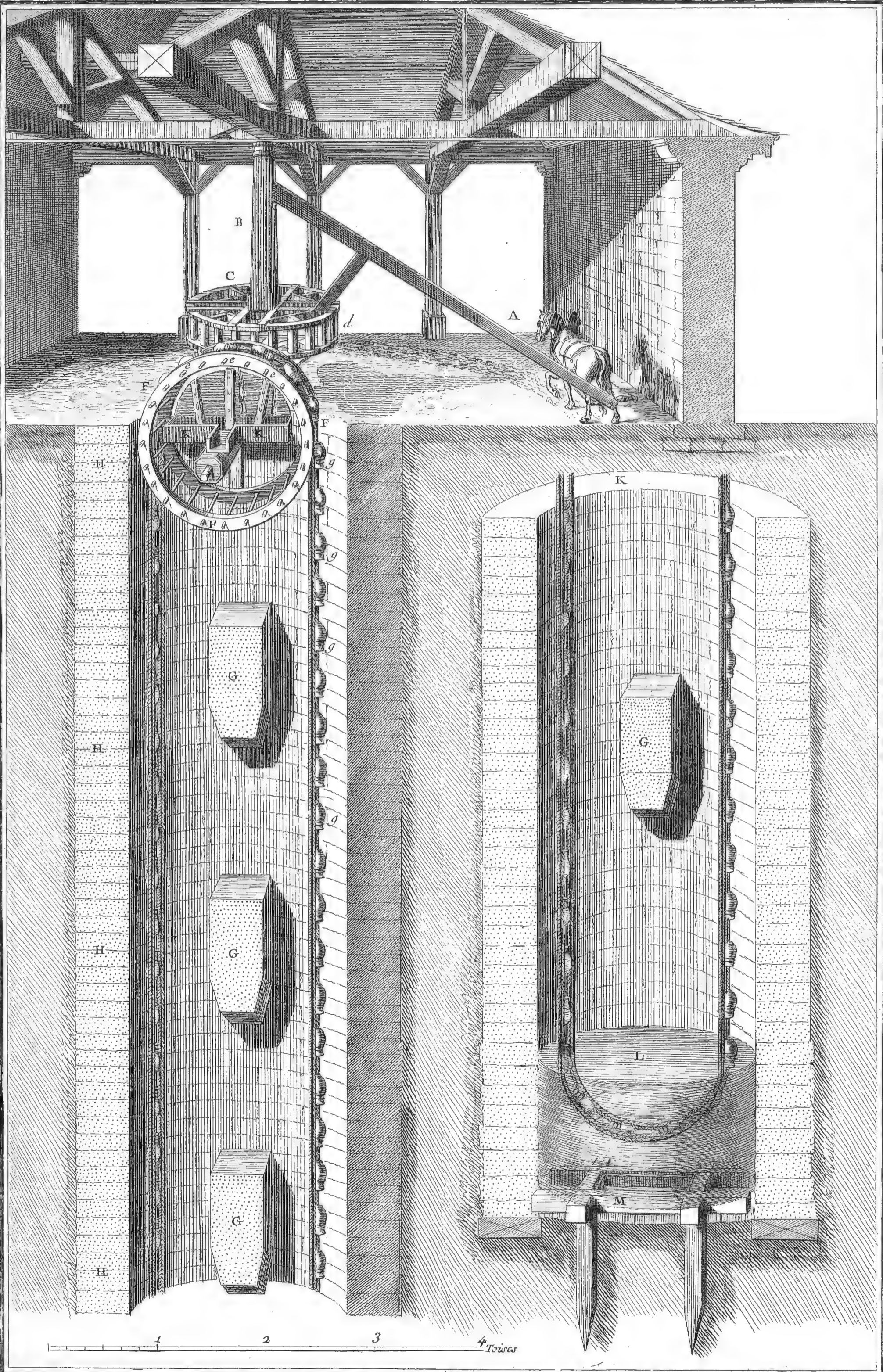
Hydraulique, Noria.
