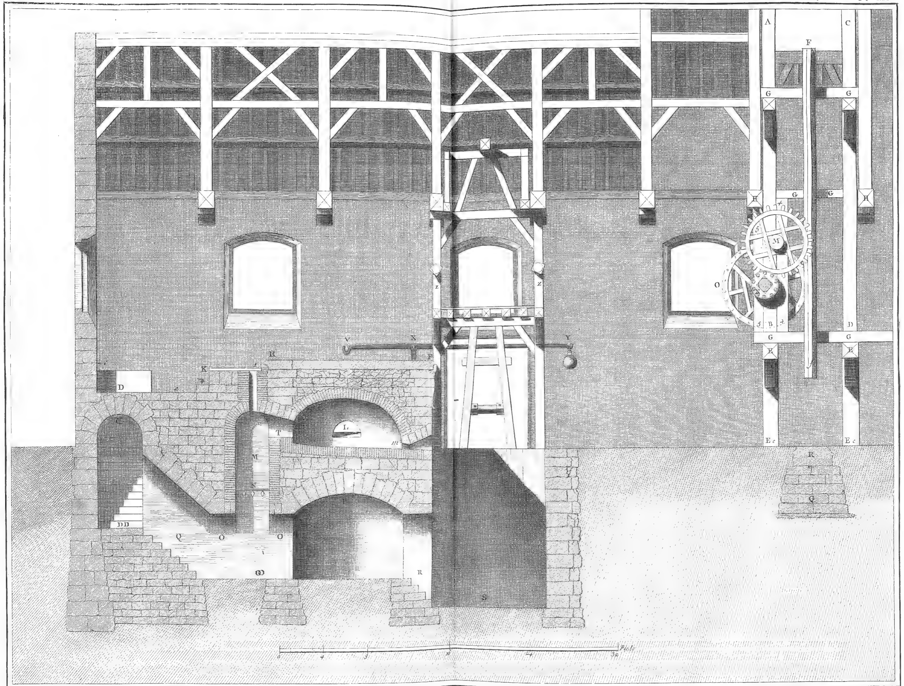
Fonte des Canons, coupe Longitudinale du Fourneau par sa Chauffe, coupe du Bessroy au dessus de la Fosse, et coupe de l'Alzoir.
