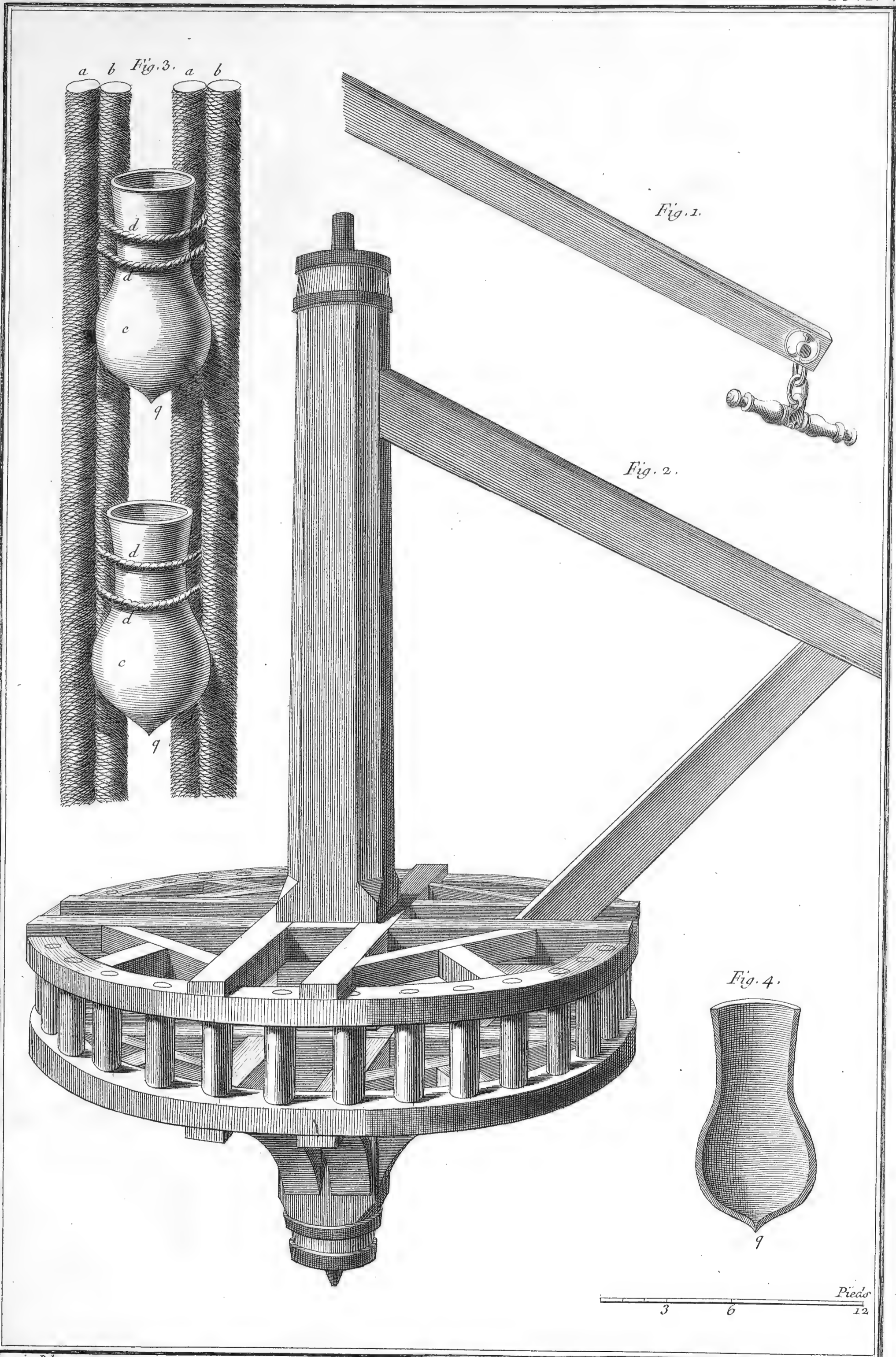
Hydraulique, Noria.
