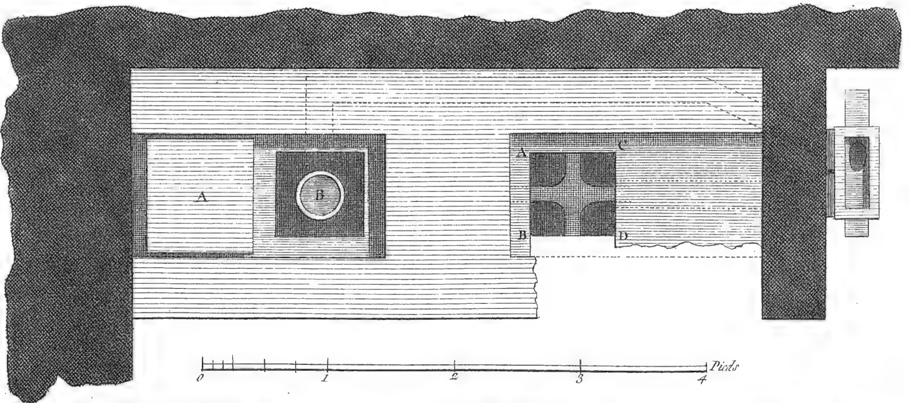
Fondeur en Sable.
