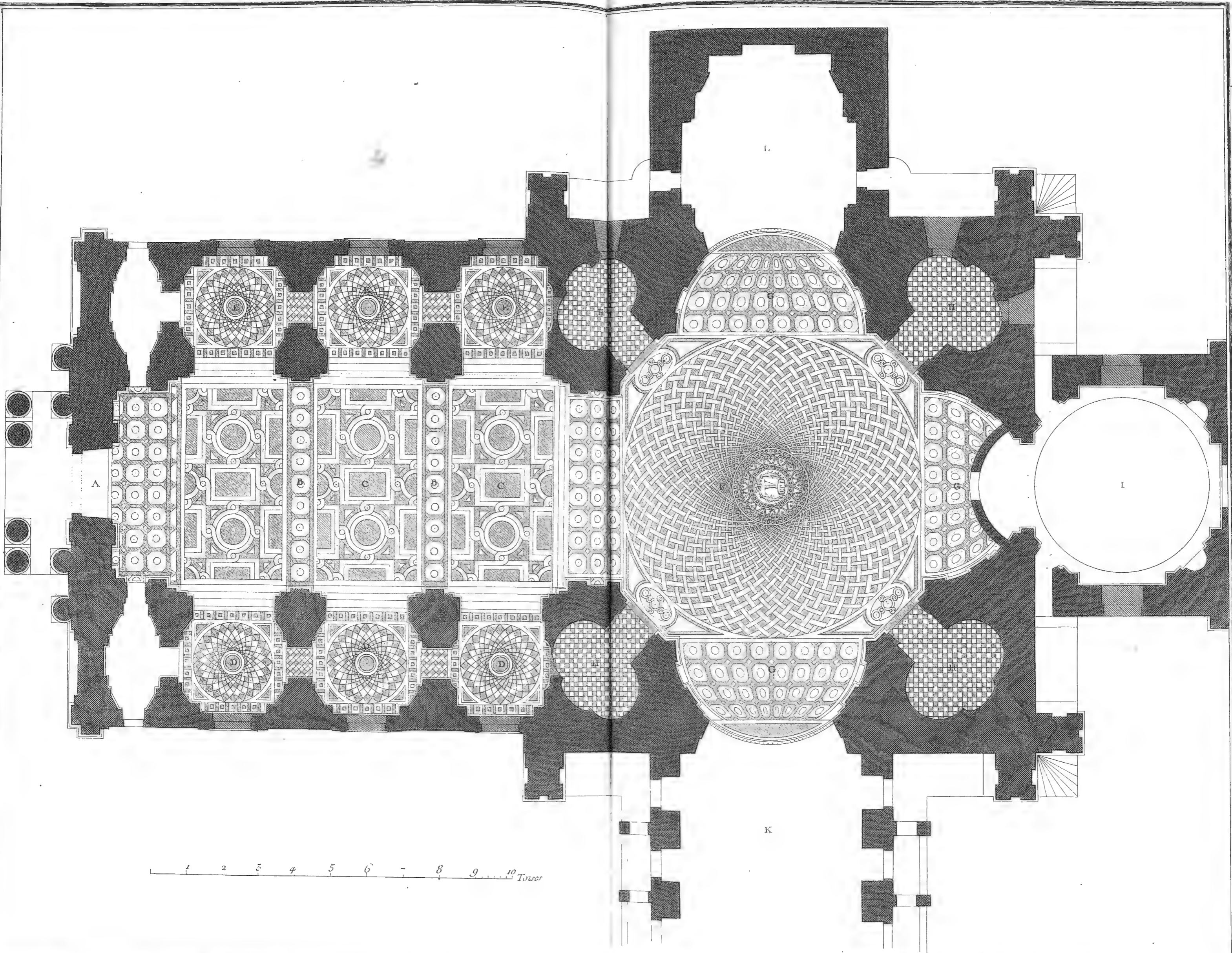
Marbrerie, Plan du pavé du Val de Grace.
