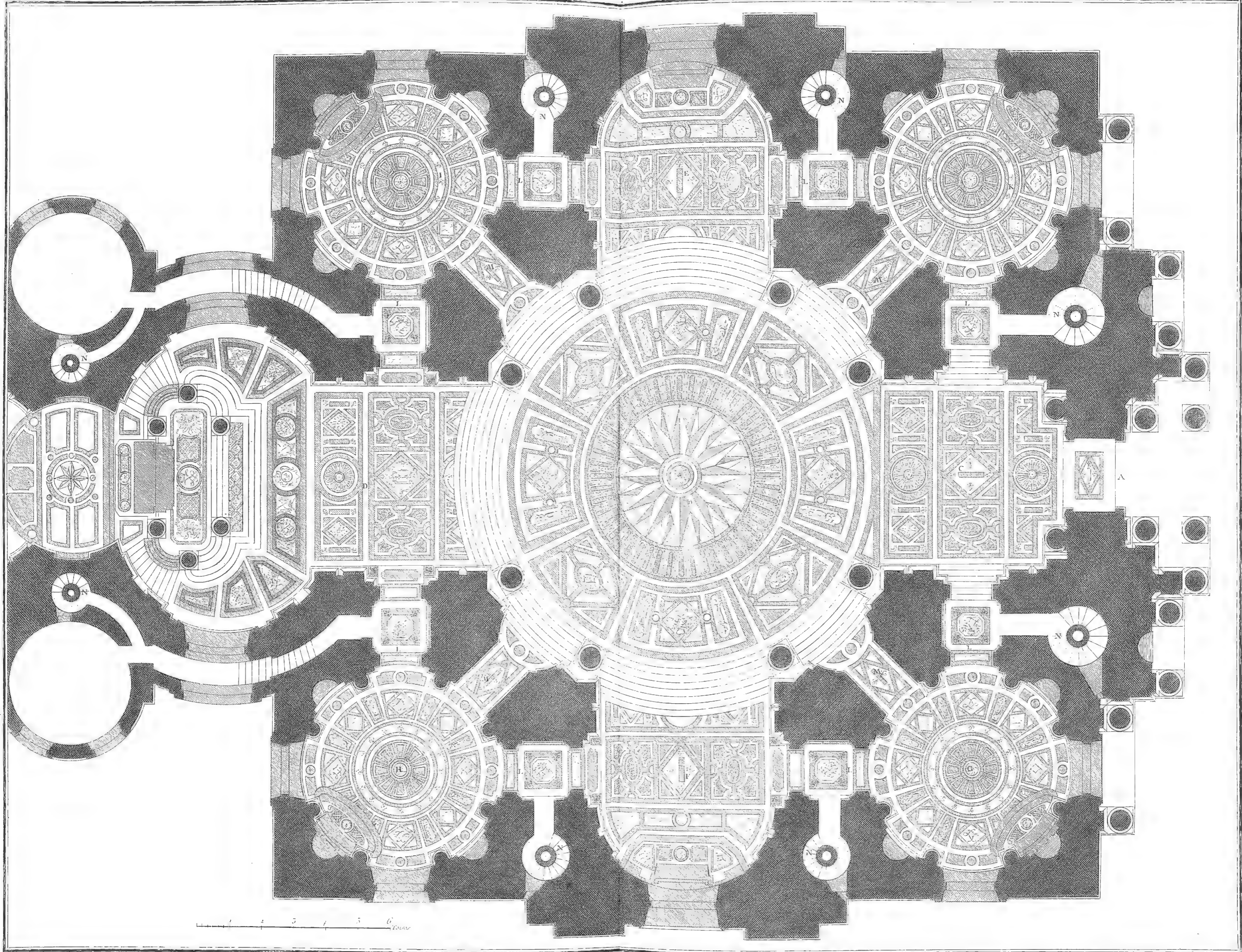
Marbrerie Plan du pavé compris sous le Dome des Invalides.
