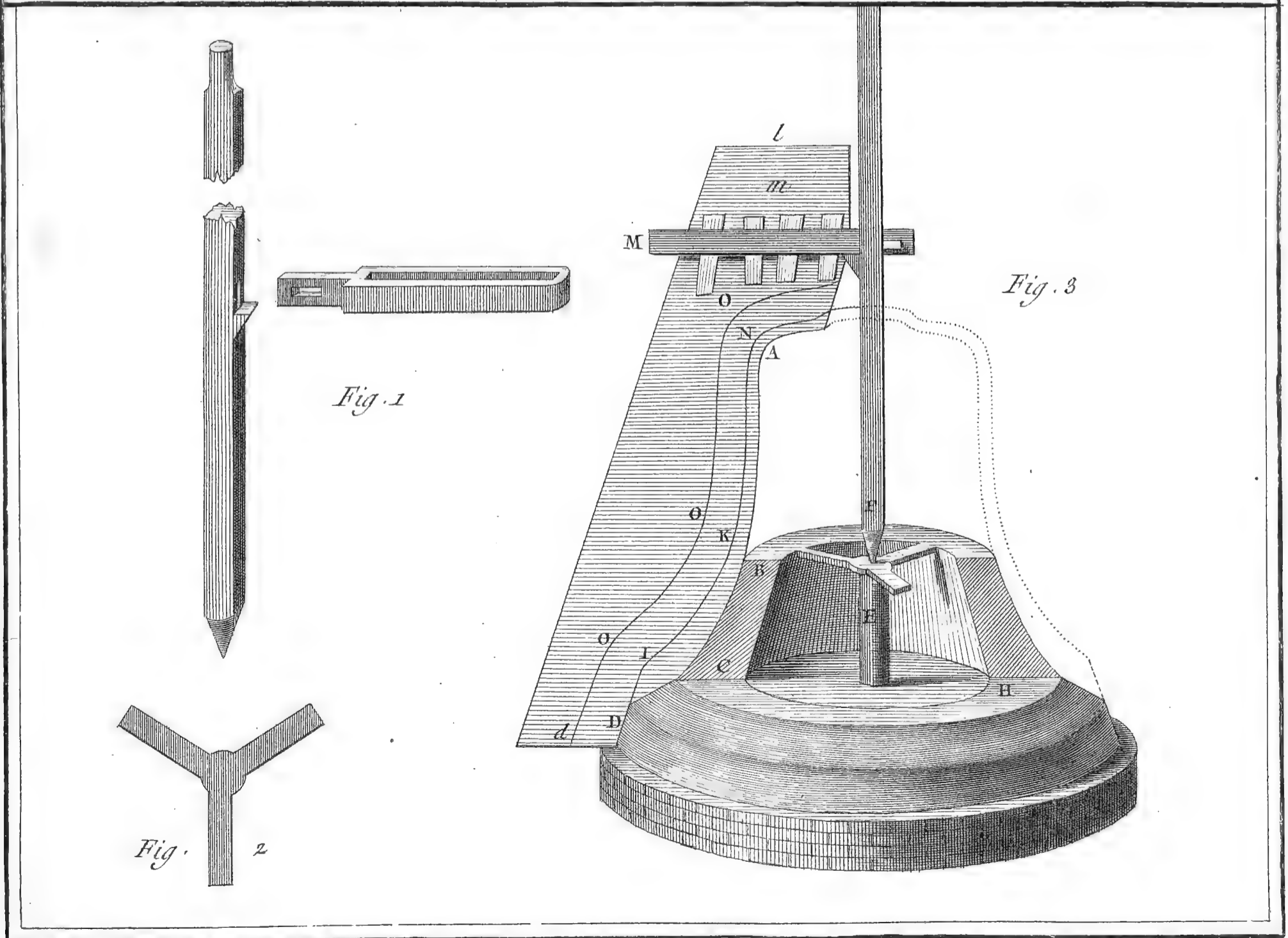
Fonte des Cloches, Fabrication du Moule.
