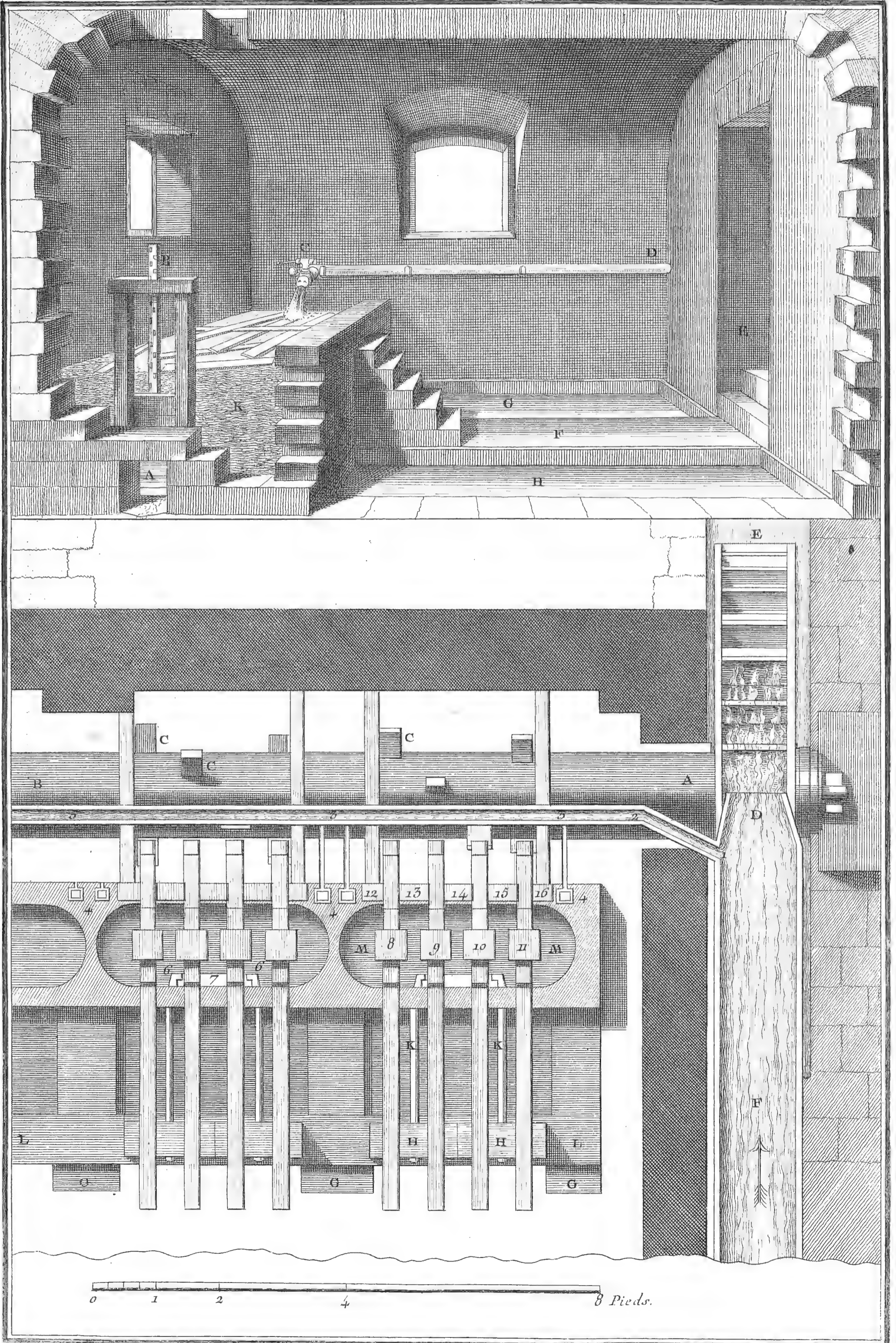
Papellerie, Pourissoir.
