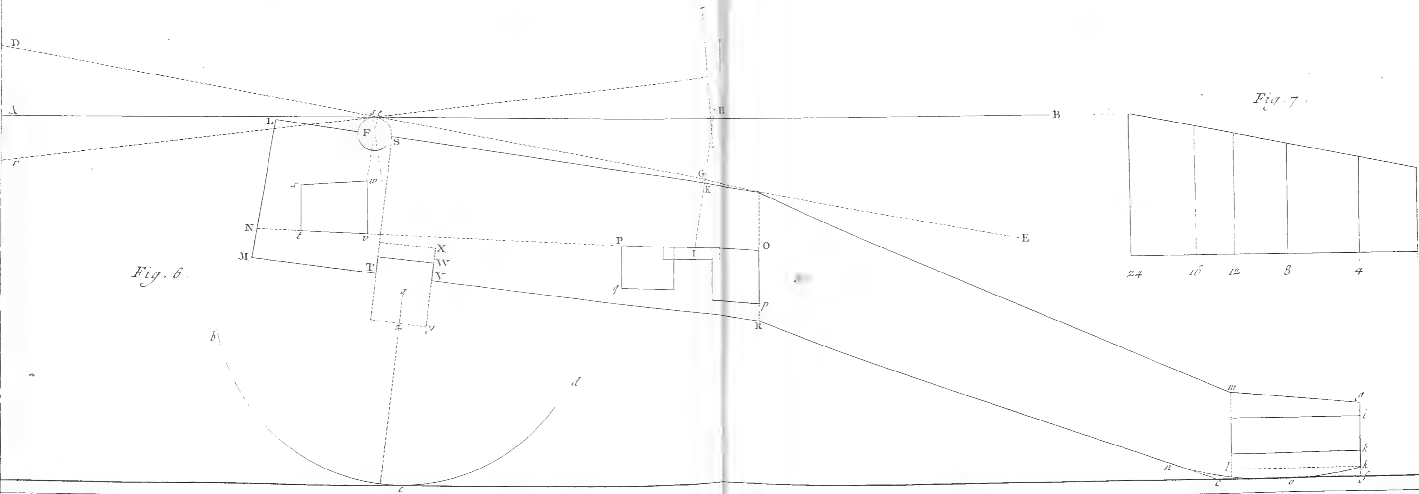
Fonte des Canons, Avant-train du Capitaine Espagnol et démonstration relative à l'art de Pointer?
