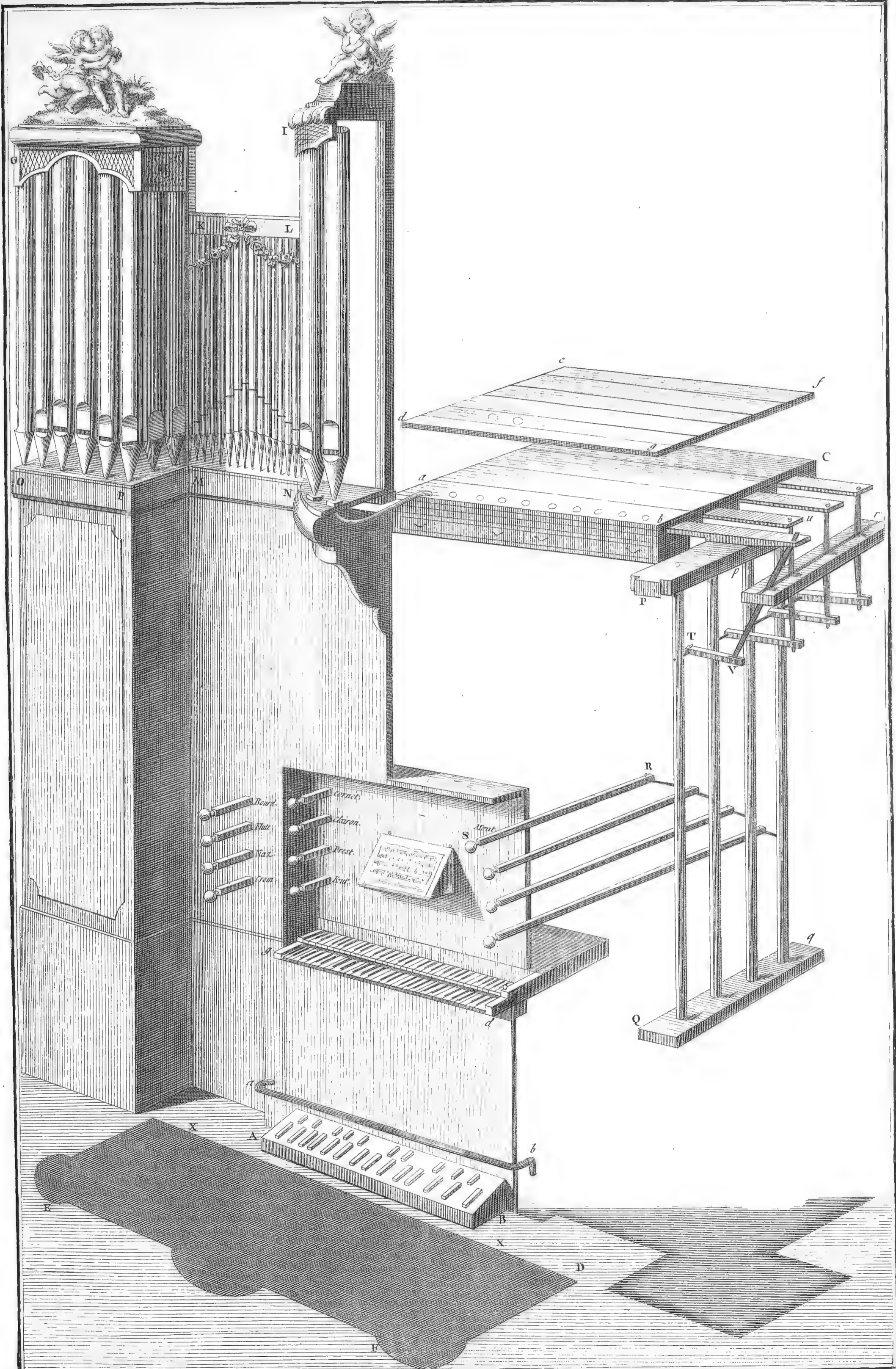
Lutherie, orgues.
