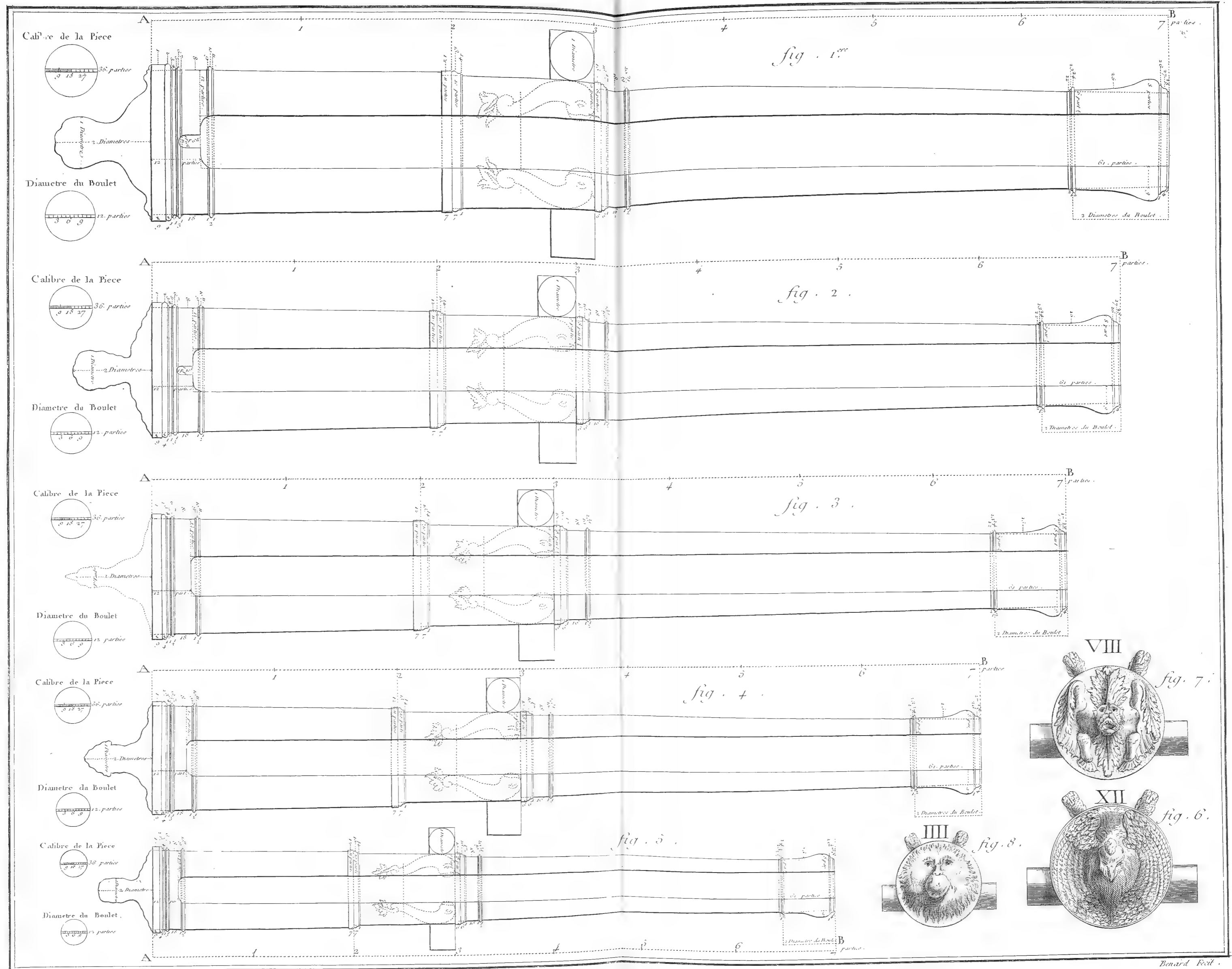
Fonte des Canons, Epures des Cinq Calibres de l'Ordonnance.
