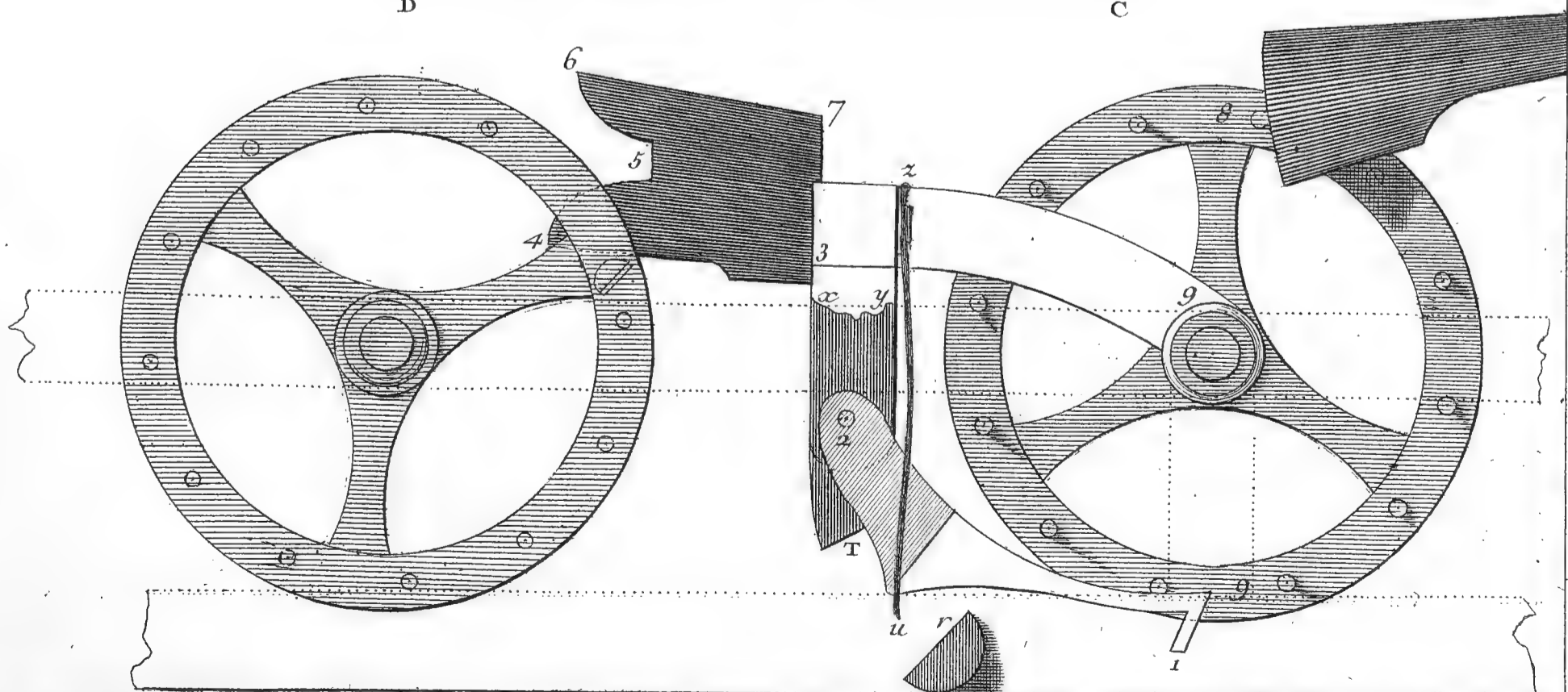
Algebre et Arithmetique. Machine Arithmetique de Pascal.
