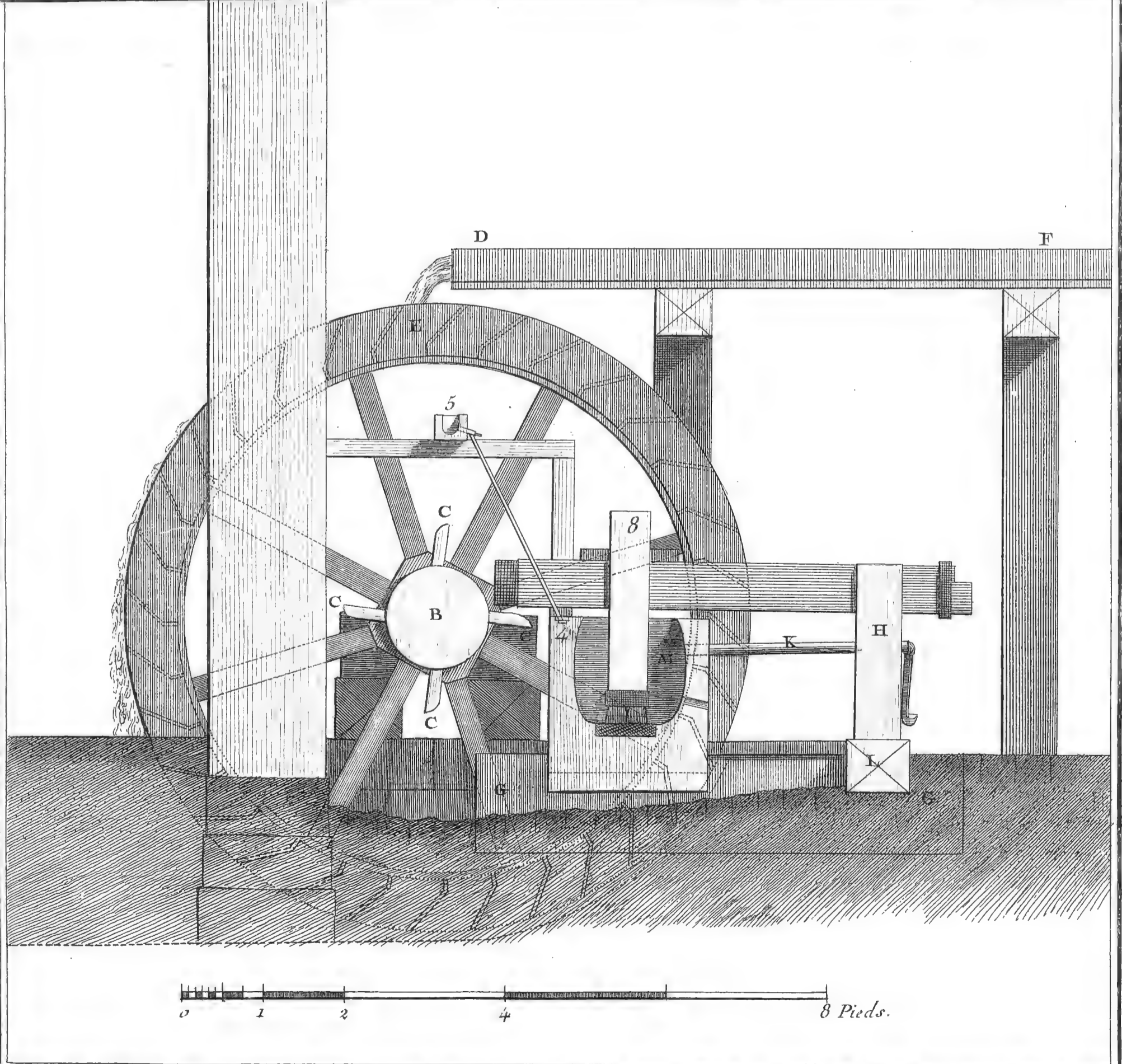
Papetterie, Dérompoir.
