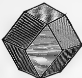
RHOMBIC DODECAHEDRON.
