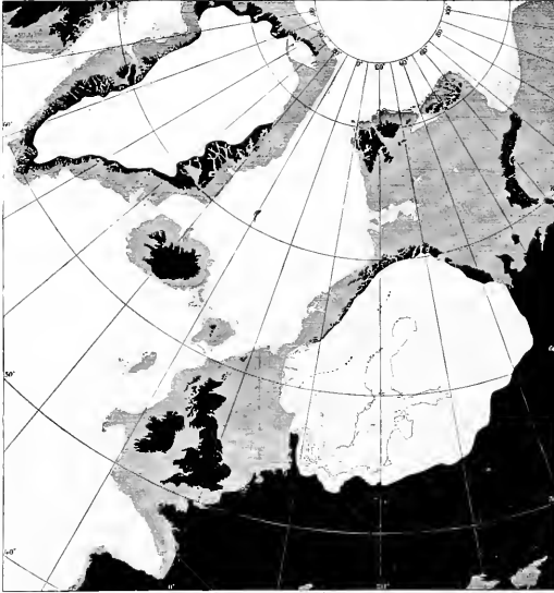
Fig. 3. Karte von Nordwesteuropa, teils die Verbreitung des Eises in der letzten Eiszeit (nach USSING), teils, des Vergleiches wegen, die jetzige Verbreitung des Landeises auf Grönland, teils die Meeresgebiete, die über 400 (gestrichelt) bzw. 600 (punktirt) m Tiefe liegen (nach NANSEN) zeigend. Die gebrochene Linie in Skandinavien bezeichnet die Eisscheide.
