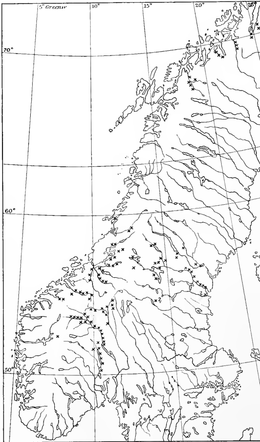
Fig. 19. Karte der beiden Verbreitungsgebiete von Myricaria germanica (x) in Skandinavien. In das zentralskandinavische Gebiet hat sich der Strauch wahrscheinlich aus den Gebirgen Norwegens an den Quellengebieten und dem Stromsystem der Ängerman- und der Indalsälk entlang bis an das Mündungsgebiet der letzteren verbreitet; im Nordnorwegischen nur in das Küsten- und Alpengebiet. Das Vorkommen in Norwegen nach ANDR. M. HANSEN.
