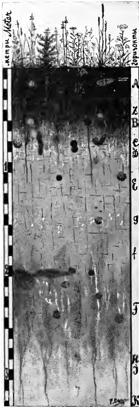
Fig. 2. Ein Durchschnitt durch schwarzen Steppenboden. Die schwarzen Flecke im Untergrunde sind von schwarzem Boden angefüllte Gänge von wühlenden Steppentiere. Die bei 2 Meter beginnenden dunklen Streifen sind von oben eingeschwennter Humus. Die kleinen weißen Punkte und Streifen sind Kalkkonkretionen (Gouvern. Woronesch).
