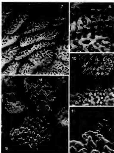
Pl. 2. — Ponthieva maculata : 7, tétraèdes de la zone intermédiaire, squamiformes, à tectum partiel discontinu à mailles polygonales, plus ou moins irrégulières \times 1\ 600 ; 8, détail du réseau au niveau du bourrelet exinal d'une tétrade \times 3\ 900 ; 9, tétrade de la zone pollinique terminale \times 5\ 500 ( tc = tectum partiel continu au niveau du bourrelet, td = tectum partiel discontinu, cl = columelles libres (disparition du tectum)); 10, tétraèdes de la zone pollinique terminale ne présentant pas de tectum, à columelles entièrement libres \times 3\ 700 ; 11, détail des têtes de columelles de la zone pollinique terminale : columelles capitées ou digitées; quelques têtes voisines sont soudées entre elles, formant ainsi une ébauche de tectum \times 7\ 300 . (Clichés M.E.B. faits au Laboratoire de Géologie du Muséum.)
