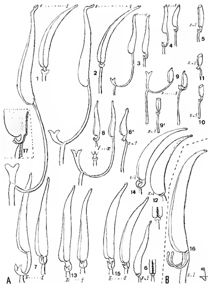
Pl. 1. — A : Étamines du type Antherotoma : Dissotis irvingiana : 1, var. alpestris (Schlieben 4329); 2, var. irvingiana (Audru 1753); 3, ( Pobéguin 1697); 4, ( Jacques-Félix 2034); 5, ( Jacques-Félix 2022); 6, ( Leuenberger 985, Mali); 7, ( Le Testu 9118). — Dissotis phaeotricha : 8, ( Trochain 1315); 8', forme osbeckioides ( Satabié 27). — Dissotis tisserantii : 9, ( Tisserant 1256); 9', forme osbeckioides ( Letouzey 5957). — Antherotoma naudinii : 10, ( Humbert 30622); A. clandestina : 11, ( Jacques-Félix 8672). — Dissotis senegambiensis : 12, ( Boudet 4761, Sénégal); 13, ( Paiva 12249, Mozambique); 14, ( W. de Wilde 9296, Abyssinie). — Dissotis densiflora : 15, ( Bobault 176). — B : Étamines du type Dissotis : 16, D. elegans ( de Witte 1202); 17, D. congolensis ( Descoings 9807). E = étamine externe; I = étamine interne. (1-16 × 6; 17 × 12).
