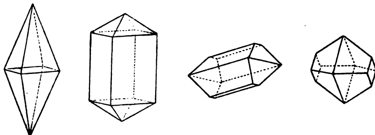
Beispiele für das rhombische System.
