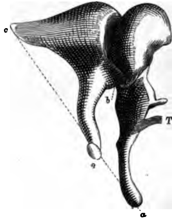
Hammer-Ambossgeleht.
