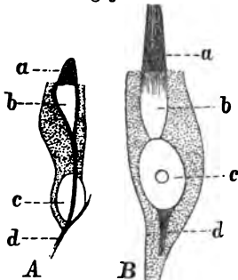
Isolierte Haarzellen.
