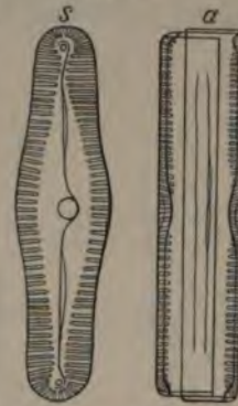
Pinnularia.
