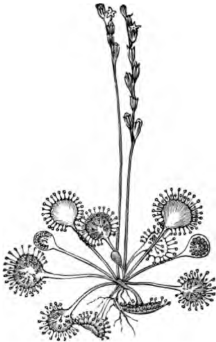
Sonnentau (Drosera).
