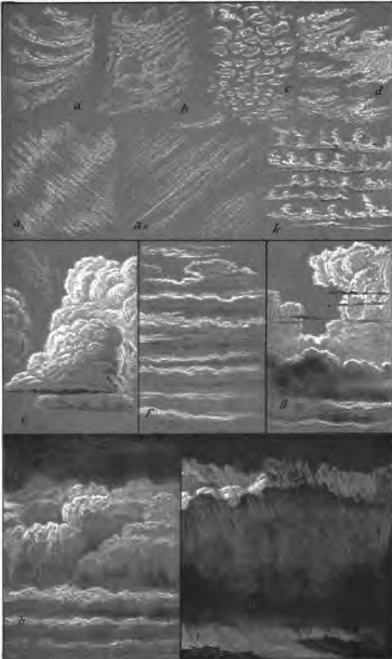
a a, u b cirrus, a , cirrus-fäden, c cirro-cumulus, d cirro-stratus, e cumulus, f stratus, g cumulo-stratus, h strato-cumulus unten Wulstcumulus, i Nimbus, k Gewitterwolke nach G. Ley
