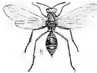
FIG. 15. Polistes bellicosus .
