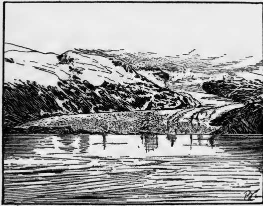
FIG. 50. SERPENTINE GLACIER.
