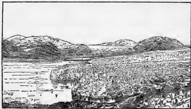
FIG. 9. MUIR GLACIER.
