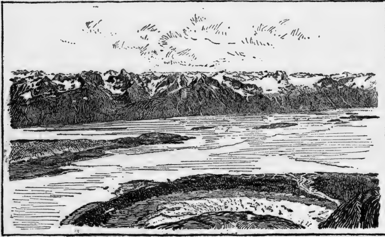
FIG. 3. DAVIDSON GLACIER.
