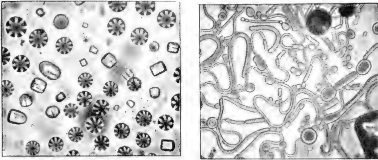
Abb. 2. „Scheinbar lebende“ flüssige Kristalle von Paraazopyrimtinsäureäthylester aus Monobromnaphthalin.
