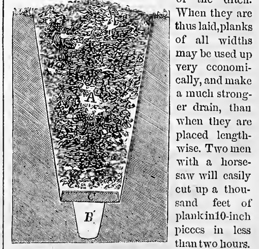
Fig. 1.—PLANK DRAIN.
