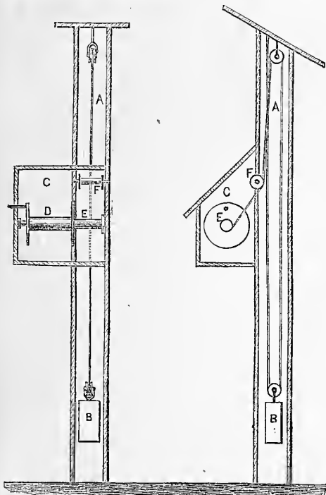
Fig. 1.—FRONT. REEL. Fig. 2.—SIDE.
