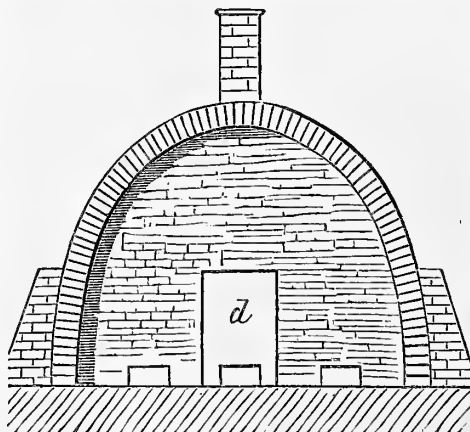
Fig. 2.—PERMANENT TILE-KILN.
