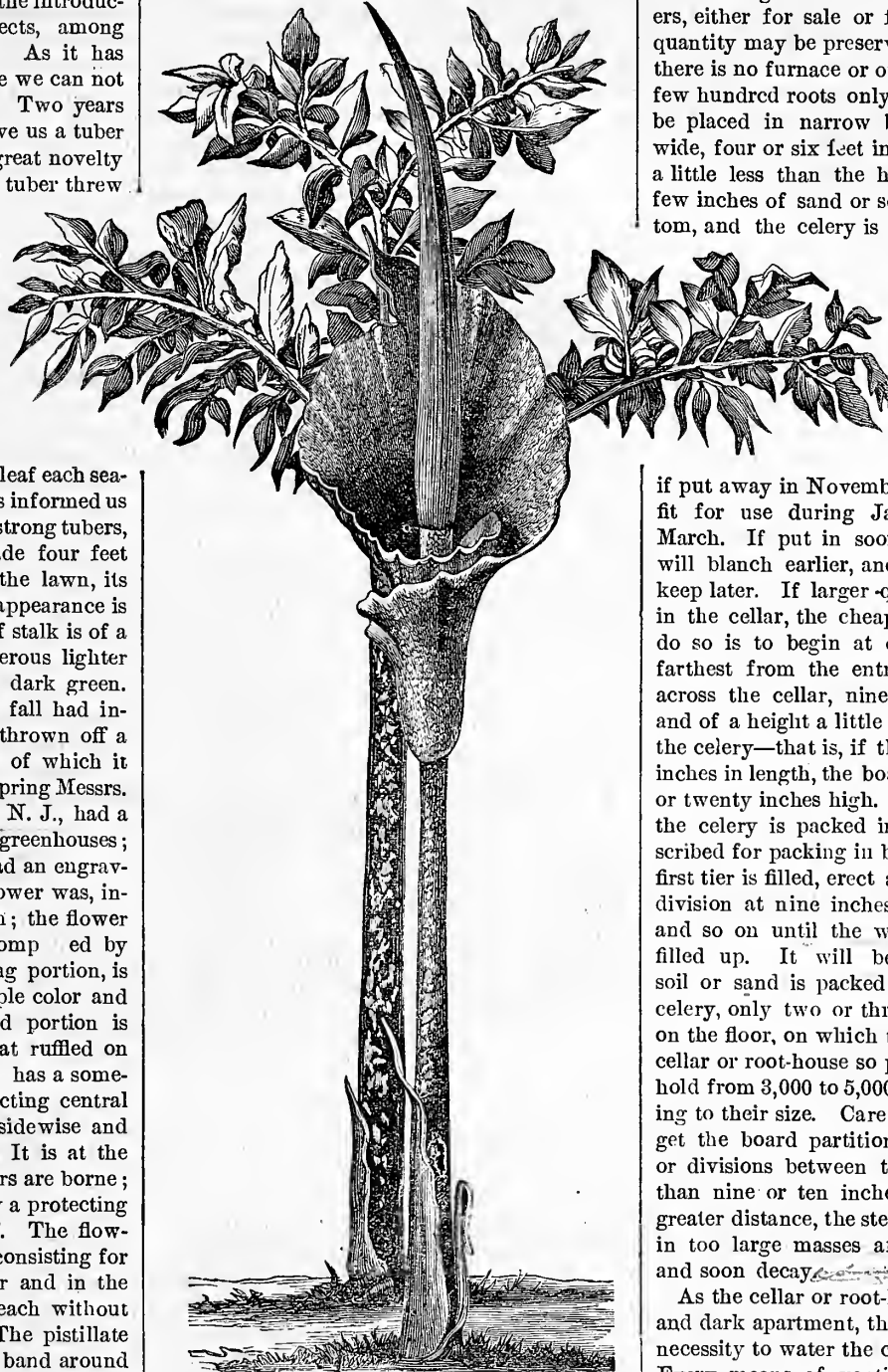
AMORPHOPHALLUS RIVIERI.
