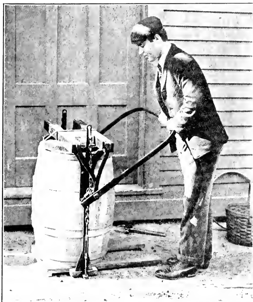
LEVER BARREL PRESS
