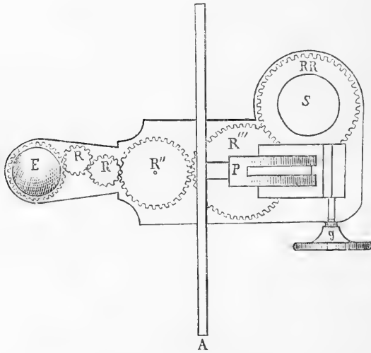
A. Seccion horizontal del sostén principal.—R, R', R'', R''', RR. Sistema de ruedas dentadas, de las cuales la primera engrana en un cruk.—P. Seccion horizontal de la pieza arqueada que sostiene una plancha.—E. Punto del eje óptico, alrededor del cual gira la esfera de las lentes.—S. Tornillo para centrar las preparaciones.—g. Tornillo destinado al movimiento de la pieza P.
