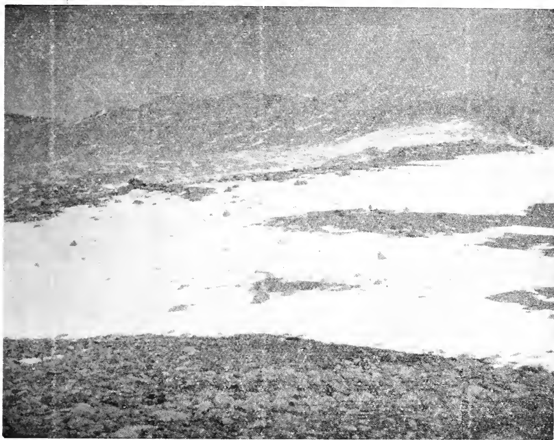
LÁMINA 5. — Parte de la plataforma cuspidal y del crestón de la cumbre del Nevado Alto Blanco, visto desde NE a 5.600 m. Fot.: Rohmeder, 1940-II-16.
