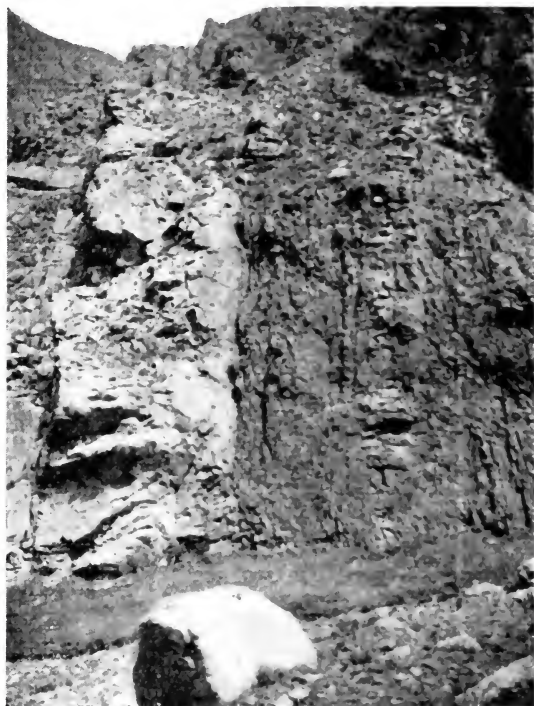
LÁMINA 8. — Contacto del granito diorítico (a la izquierda), con las rocas córneas, en el valle superior del río Remanso.
