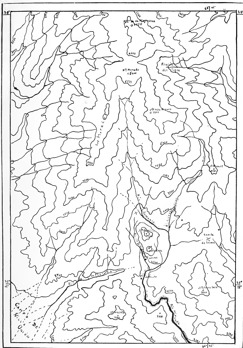
PLANO 1.— Mapa hipsométrico del Valle de Cosme (Sierra de Famatina), según el plano manuscrito n° 483 de la Sección Topográfica de la Dirección General de Minas y Geología, Buenos Aires, y observaciones propias del autor. Escala aproximadamente 1: 220.000.
