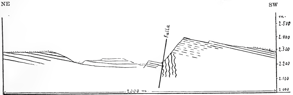
Corte geológico a través del Valle de Cosme, al noroeste de la confluencia de los Ríos Remanso y Santo Domingo.
