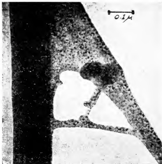
FIG. 18. — Cloruro de vinile polimerizado (aumento 100.000 diámetros). De Trans. El. Eng. , 1941, pág. 161.
