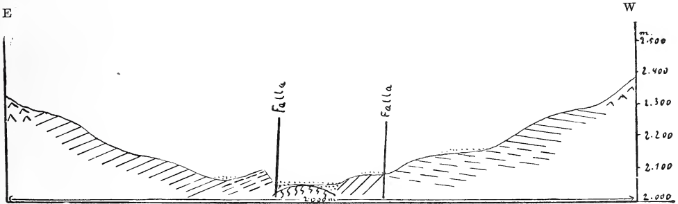
Corte geológico por el valle del Río Miranda, cerca del Puesto de Vallecito.
