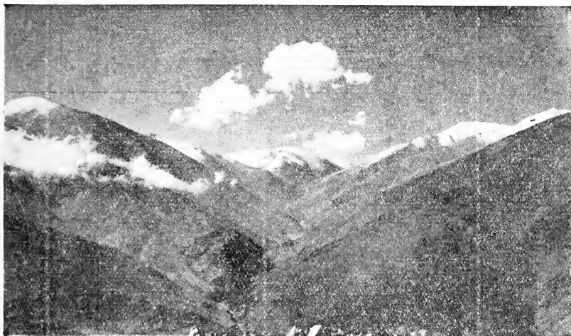
LÁMINA 1. — Valle superior del río Remanso, visto desde el S., hacia el Nevado Morado, a 3.000 m. Fot.: Rohmeder, 1940-II-18.
