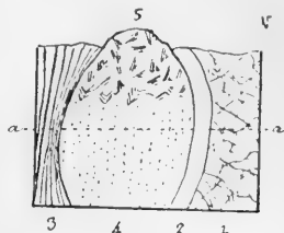
1. Roca cristalina descompuesta.—2. Pizarra carbonosa del culm.—3. Pizarras diversas del culm, trastornadas.—4. Pirita.—5. Coronamiento de limonita.
