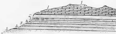
Coupe du terrain crétacé à Uña.
