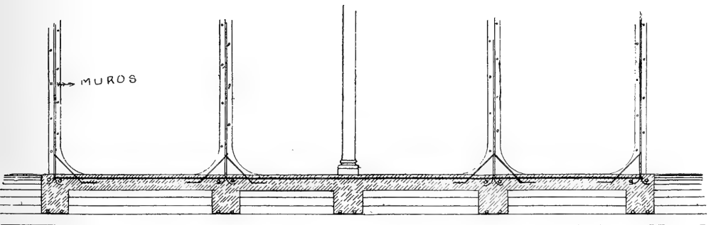
CORTE XY ~ Plataforma de base ~
