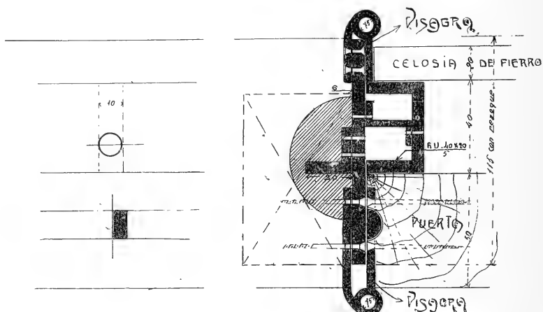
Fig. 50. — Tipo de marco de hierro
