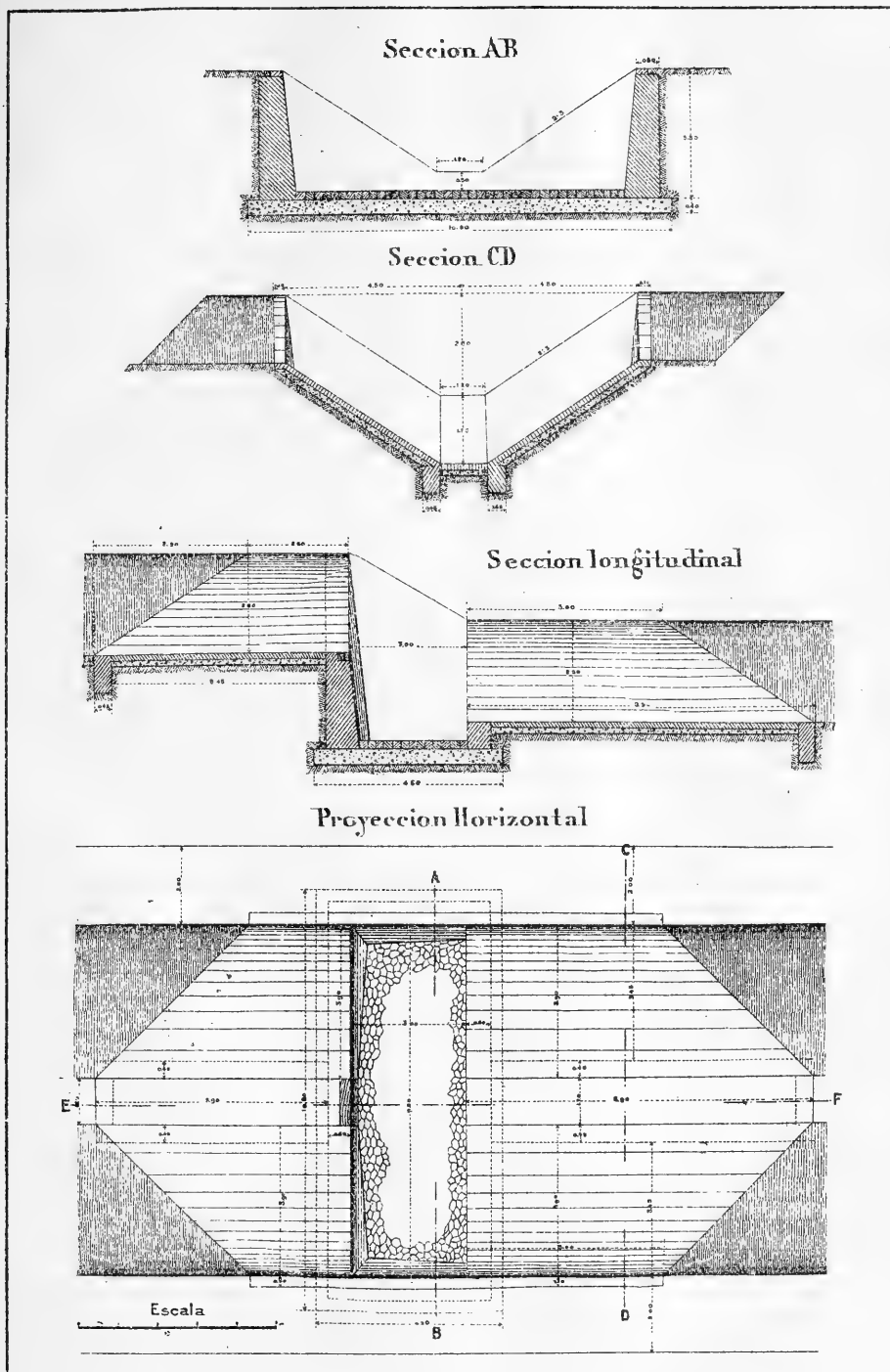
TIPO DE SALTO DE 1.75 de Altura: Hm. 27. - 42.27
