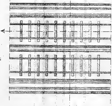
Proyeccion Horizontal
