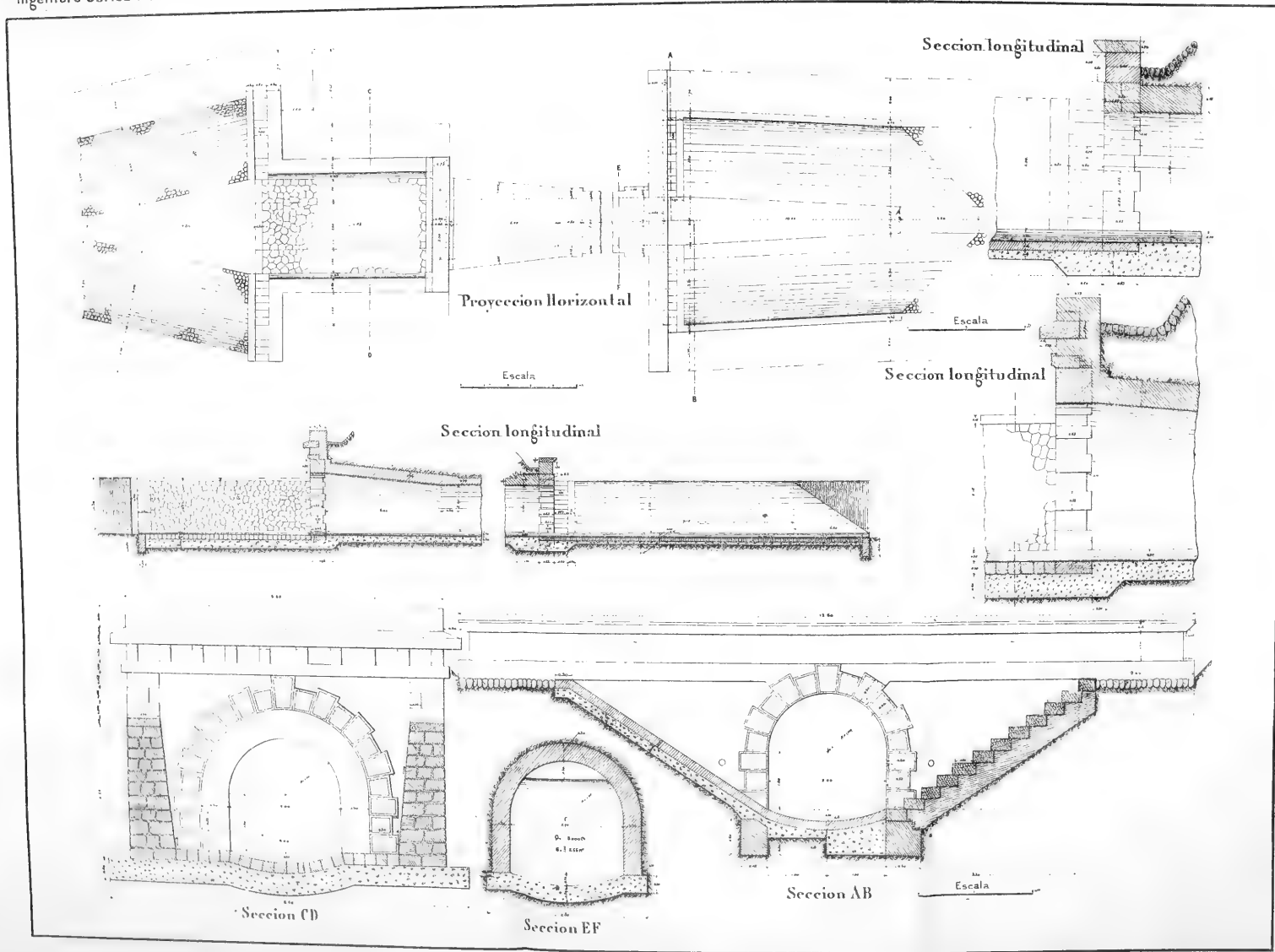
TUNEL DEL COIMENAR.
