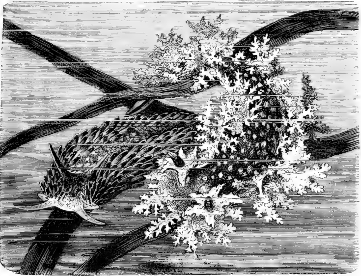
Fig. 19.— Eolis and Dendronotus .
