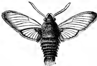
Fig. 27.- Bee Hawk Moth.
