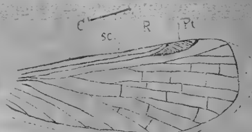
Fig. 6. — Orthophlebioides reticulatus HANDL. 55 — Lias d'après A. HANDLIRSCH (montre que le pterostigma dépend de la radiale).
