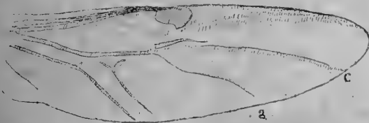
Fig. 5. — Aile d' Apatetica (d'après BONDRÖIT).
