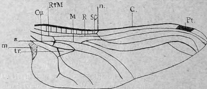
Fig. 1. — Aeschna affinis VANDERL. 2/1 (aile postérieure) d'après K. REZSÖ. C = costale, sc = sous-costale, R = radiale, M = médiane, Cu = cubitale, a = arcus, n = nodus, m = membranula, tr = triangle, Pt = pterostigma.
