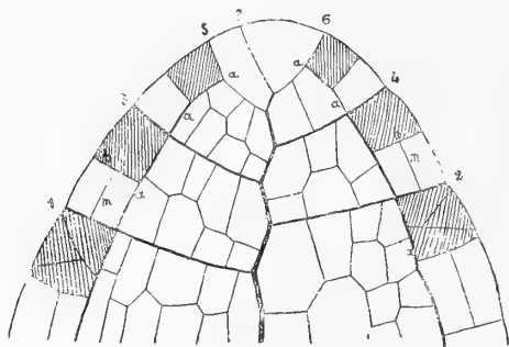
Fig. 1. — Sommet de la tige du Pinus rigida . Figure théorique.
