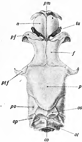
Fig. 1. Cranium cerebrale von Vipera Ursinii BONAP. von oben. Adultes ♀ aus Laxenburg. Vergr. 4. co = der dreitheilige Condylus occipitalis, f = Frontale, n = Nasale, ol = Occipitale laterale, op = Opisthoticum, os = Occipitale superius, mit dem Epitoticum verschmolzen, p = Parietale, pf = Præfrontale, pm = Præmaxillare, po = Prooticum, ptf = Postfrontale, tu = Turbinale.
