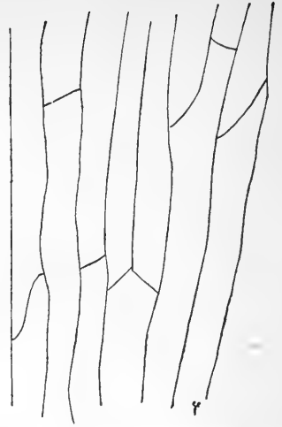
Fig. 2. — Frammento dello stesso strato cellulare raffigurato in fig. 1, ma prelevato in parte distale alla apertura intrastilare. (Ingr. 20 diam.)
