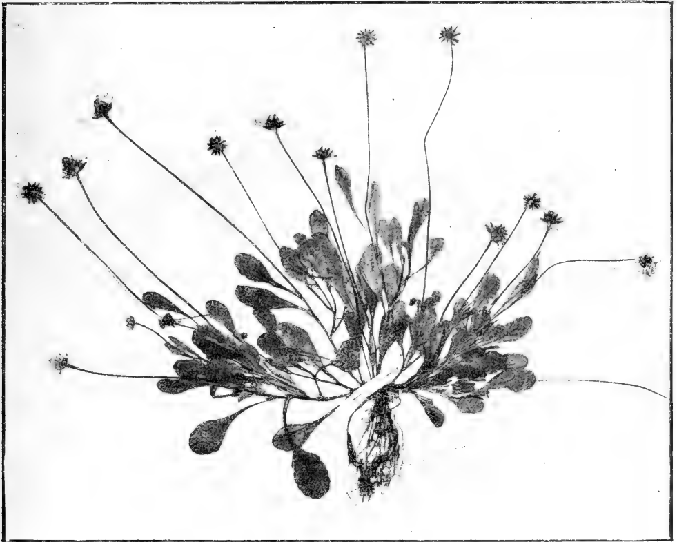
Fig. 8. — Un individuo della generazione F_2 ( B. perennis × B. annua ) × ( B. perennis × B. annua ) ( \frac{1}{3} grand. nat.).
