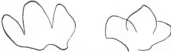
Fig. 5. — A sinistra porzione di calice aperto di C. Cesatiana a destra di C. pentagona . (Ingr. circa 10 volte).
