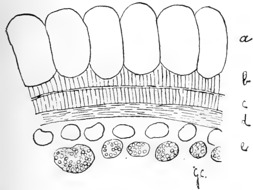
Fig. 12. — Sezione attraverso il tegumento seminale di C. europaeae . a) epidermide; b) strato di cellule palizzata; c) id.; d) perisperma; e) strato proteico e strato amilaceo. (Ingr. diam. 210 circa).
