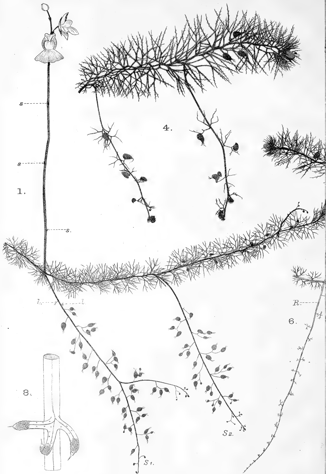
GLÜCK — UTRICULARIA.
