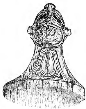
FIG. 27.—Head-ornament of Fig. 24. \frac{1}{8} .
