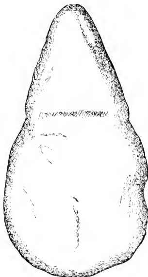
FIG. 16.—Grooved celt. \frac{1}{2} .
