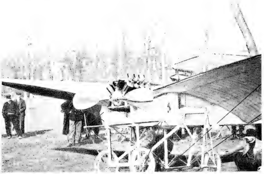
1. Antoinette monoplane with Lavavasseur Antoinette engine, 1909.
