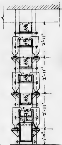
SECTION A-B.
