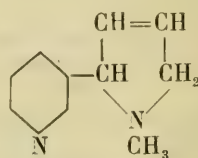
IV. Nicotéine.
