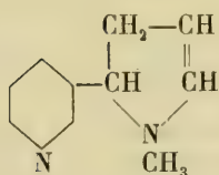
III. Déhydronicotine.
