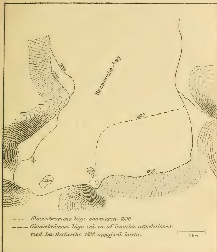
Modifications éprouvées par les glaciers de l'Est et de la Pointe des Renards, de 1838 à 1890. Carte levée par J. A. Björling (Extrait de G. Nordenskiöld, Redogörelse för den svenska expeditionen till Spetsbergen 1890 in Bihang till K. Svenska Vet-Akademi Handlingar , 1892).
