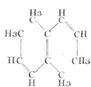
10. Naphthaterpène. C 10 H 16 .
