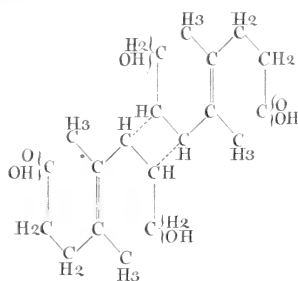
11. C 20 H 32 O 6 .
