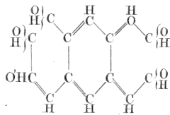
17. Acide angélicique. C 5 H 8 O 2 .
