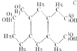
21. Acide quinqtannique. C 14 H 16 O 7 .
