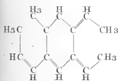
15. Anthraterpène. C 14 H 18 .
