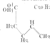
17. Acide angélicique. C 5 H 8 O 2 .
