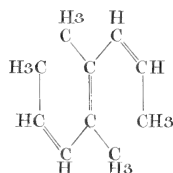
4. Noyau naphthalinique ouvert, Terpène. C 10 H 16 .
