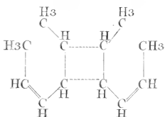
2. Dibenzoterpène. C 12 H 20 .
