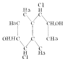
8. Dichlorhydrine de terpène. C 10 H 16 ? (Cl.OH)
