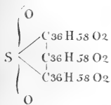
9. Combinaison sulfurique. C 36 H 58 O 2 S.
