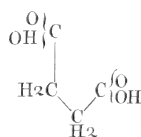
7. Acide propionique. 8. Acide succinique. C 3 H 6 O 2 . C 4 H 6 O 4 .
