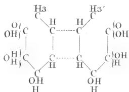
6. C 12 H 20 O 8 .
