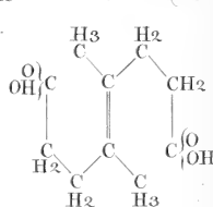
18. Acide camphorique. C 10 H 16 O 4 .
