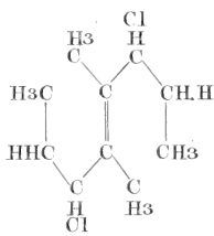
7. Dichlorhydrate de terpène. C 10 H 16 ? (HCl)
