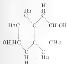
6. Terpène. C 10 H 16 ? (H.OH)
