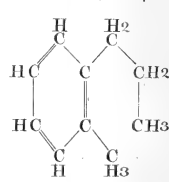
13. Cymol. C 10 H 14 .
