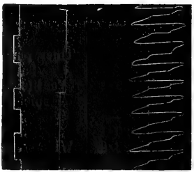
Curve IV. Inspirationsluft = 11.4 Proc. CO 2 —23.1 Proc. O. In 6" = 200 ccm = 2000 ccm pro Min. u. 9 Resp. = 90 pro Min.; 22.2 ccm pro Resp.
