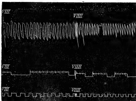
Curve VIII. In 15 Sec. 200 ccm und 17 Resp. 800 ccm pro Min.; 11·8 ccm pro Resp. Widerstand geringer als bei V. 8·2 Proc. CO 2 .
