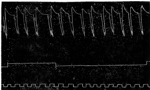
Curve VII. Voit's Ventile 12·4 Proc. CO 2 , 500 ccm pro Min.; 25¼ Resp. pro Min.; 20 ccm pro Resp.
