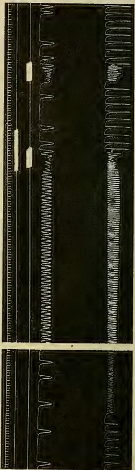
Fig. 19. Alleinige Triichterfaradisation (0 mm R. A. u. 7" Dauer) hat keine Nachwirkung; bei gleichzeitiger Vagusreizung (0 mm R. A. u. 16 1/2" Dauer) tritt eine hochfrequente, automatische Vorhoffibrillation (fast 5 Min. andauernd) und eine weniger frequente Kammerpulsation (98" lang während) auf. Später wieder normale Herzschlagfolge, abgesehen vom partiellen Block, der schon vor der ersten Reizung bestand. Die Kurven zeigen nur Beginn und Schluß der Erscheinungen; (spontan schlagendes, atropinisiertes Herz).
