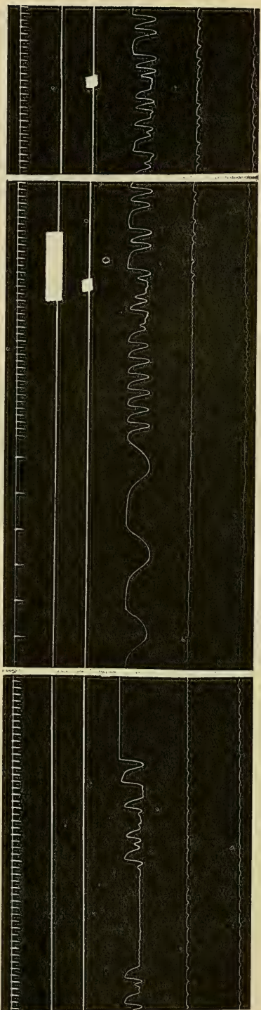
Fig. 20. Faradische Reizung der Trichtergegend (30 mm R. A. u. 1 3/4" Dauer) bewirkt nur nachträglich einzelne Extrasystolen, bei gleichzeitiger Vagusreizung (0 mm R. A. u. 10" Dauer) tritt an der Kammer kurz dauerndes Wühlen, am Vorhof gegen 2 Min. anhaltendes Nachwühlen auf. Sinusschlagfolge (oberste Kurve) bleibt unverändert; die Kammer schlägt während des Vorhofwühlens vom Sinus vollkommen unabhängig in selbständigem Rhythmus automatisch. Später wieder normale Vorhoffähigkeit, an der Kammer spontanes Wühlen bzw. doppelte Extrasystolen. Die Figur zeigt nur Beginn und Ende der Erscheinungen, zum Teil bei größerer Geschwindigkeit registriert; (spontan schlagendes Herz).
