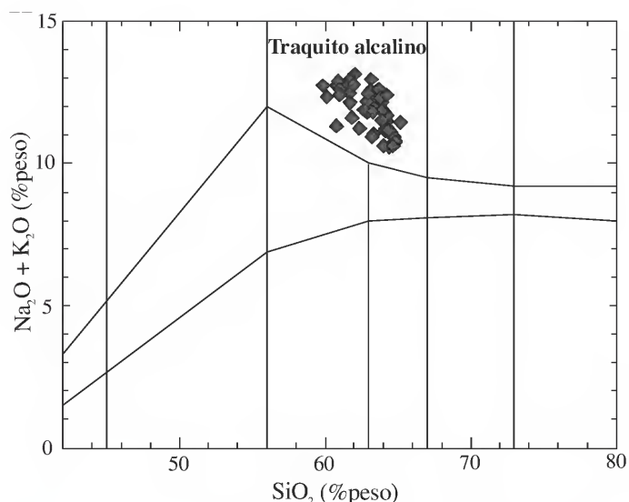
Fig.5- Diagrama \text{SiO}_2 \times (\text{Na}_2\text{O} + \text{K}_2\text{O}) para classificação de rochas (MIDDLEMOST, 1985) com as amostras de traquitos coletadas na área de estudo.
