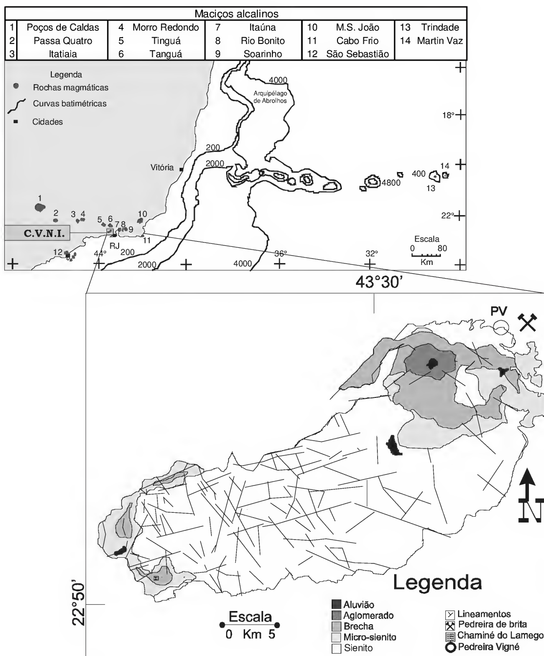
Fig.1- (a) Mapa esquemático do Lineamento Magmático Poços de Caldas-Cabo Frio; (b) Mapa de localização do Complexo Vulcânico de Nova Iguaçu (CVNI) e da área de lava da Pedreira Vigné. (modificados de KLEIN & VIEIRA, 1982; KLEIN, 1993).
