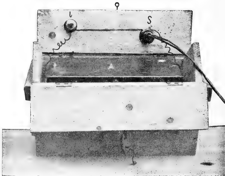
Fig. 5 a — Accumulatore (A) dentro la cassa che fa da custodia, nel cui coperchio sono l'interruttore (I) e l'attacco per la spina (S).
