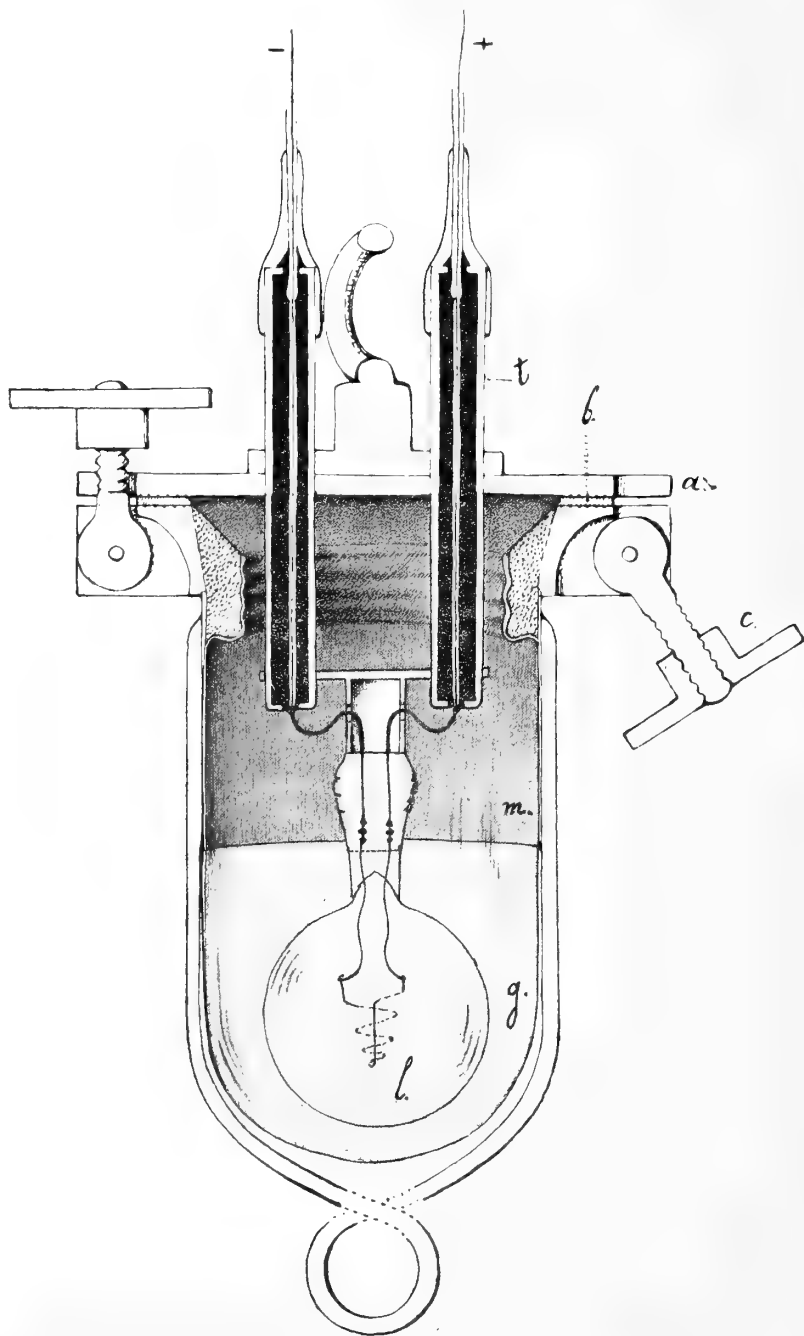
Fig. 3 a — Sezione della lampada per mostrare le diverse parti. a ) coperchio metallico, b ) striscia di guttaperga, c ) chiavarde, g ) globo di vetro, l ) lampada elettrica, m ) manicotto di ottone, t ) Tubi metallici riempiti di mastice, dentro cui passano i fili per la corrente. —, +) fili che trasportano la corrente. (Circa metà del naturale).
