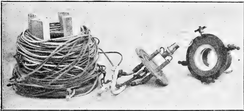
Fig. 4 a — La lampada smontata per mostrare il coperchio ed il portalampada con i fili ed il cavo avvolti su l'argano.
