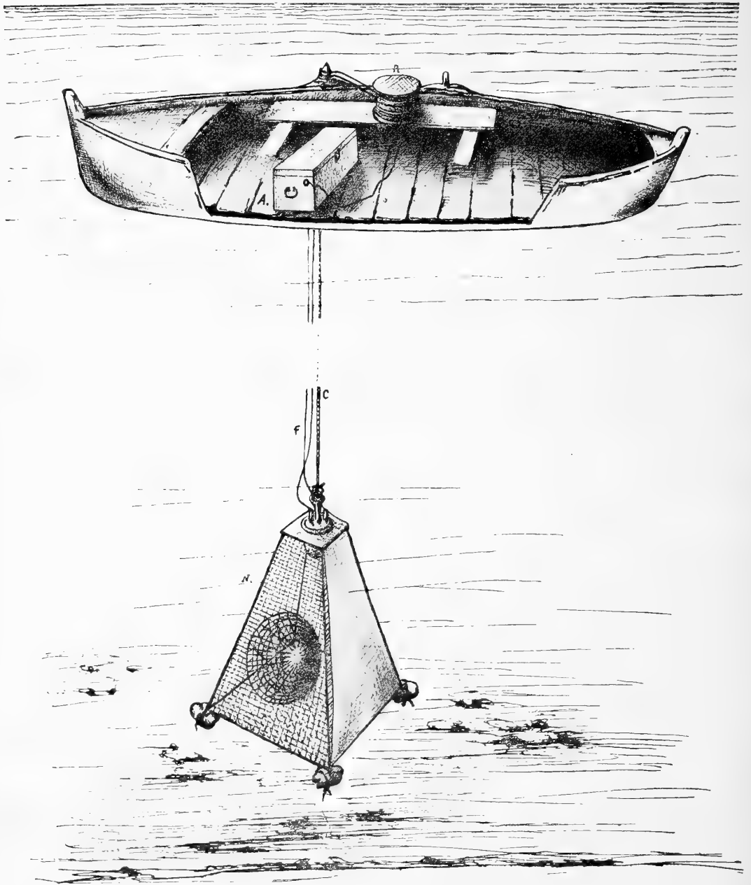
Fig. 1 a — Dispositivo per la pesca con luce subacquea. Nella barca si trovano l' Accumulatore A e l' Argano R con il filo conduttore della corrente. N ) Nassa , che poggia sul fondo marino, F ) Fili conduttori, C ) cavo di rinforzo.
