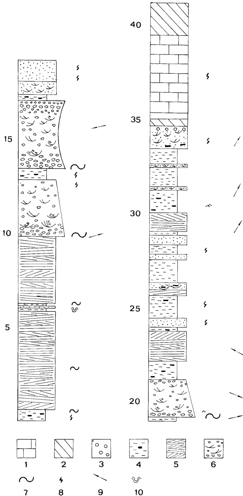
Fig. 2. — Sezione stratigrafica misurata. 1) Biomicriti ad Antrachoporella ; 2) Biomicriti ad Epimastopora ; 3) calcareniti a Fusuline ; 4) Peliti bioturbate con frustoli carboniosi; 5) arenarie con stratificazione incrociata a basso angolo; 6) conglomerati; 7) superficie erosiva; 8) bioturbazione; 9) paleocorrenti; 10) pseudo-budinaggio.
