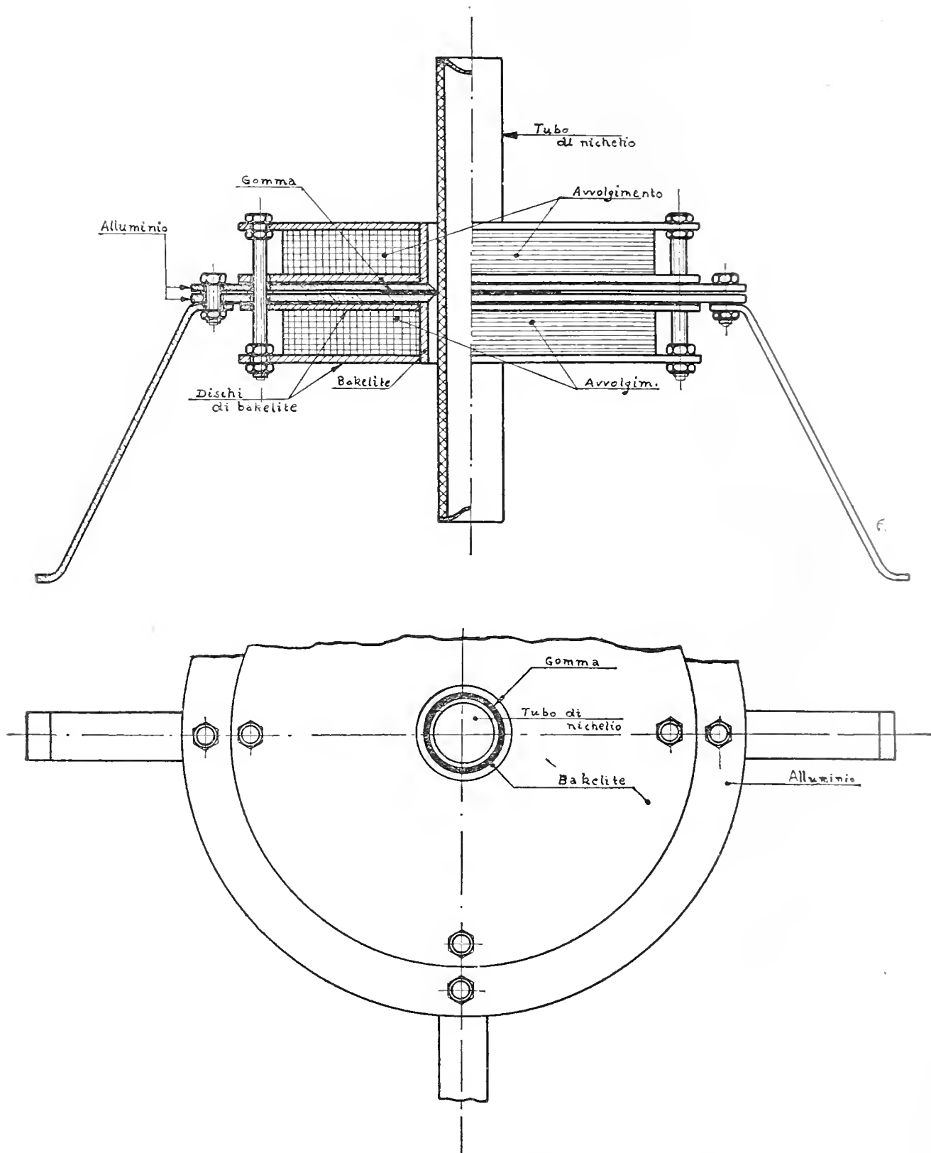
Fig. 3 — Complesso magneto-oscillante.
