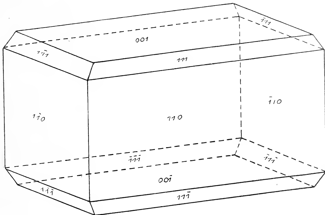
Fig. 4 — Baritina. Combinazione \{001\} \{110\} \{111\}
