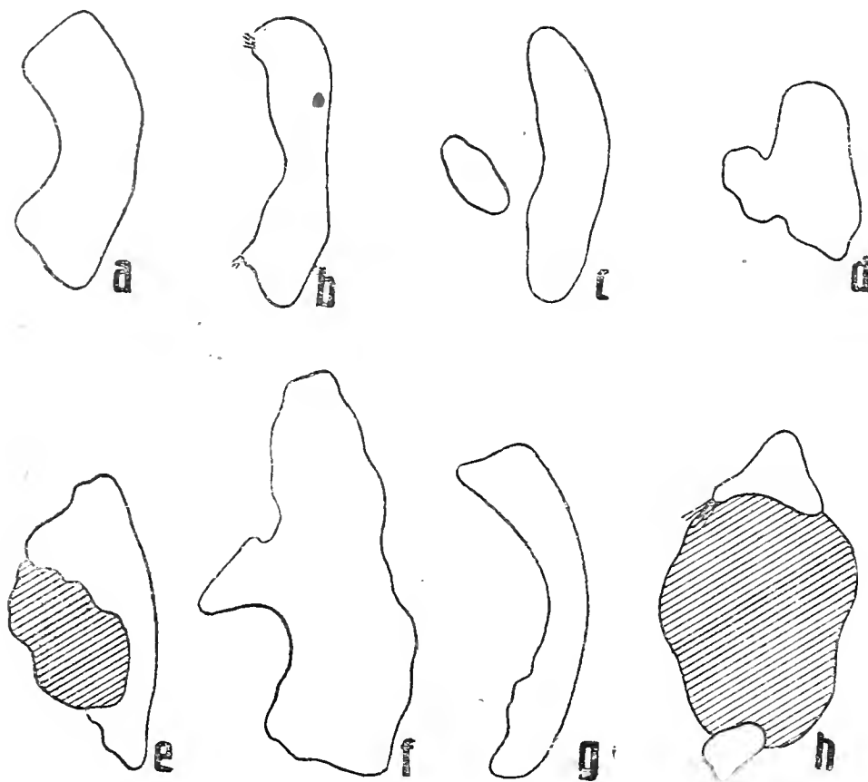
Fig. 2. — Contorno di occhio: a , B\ otri/otri - b , B\ otri/otri (con ciuffetti di peli) - c , B\ otri/otri (gli ommatidi sono raggruppati in due aree) - d , B\ otri/otri (particolarmente irregolare) - e , B\ otri/otri (l'area tratteggiata indica un'escrescenza priva di ommatidi) - f , B/+otri/otri - g , B/B\ otri/otri - h , B/B\ otri/otri (gli ommatidi sono divisi in due aree separate da una escrescenza). \times 78
