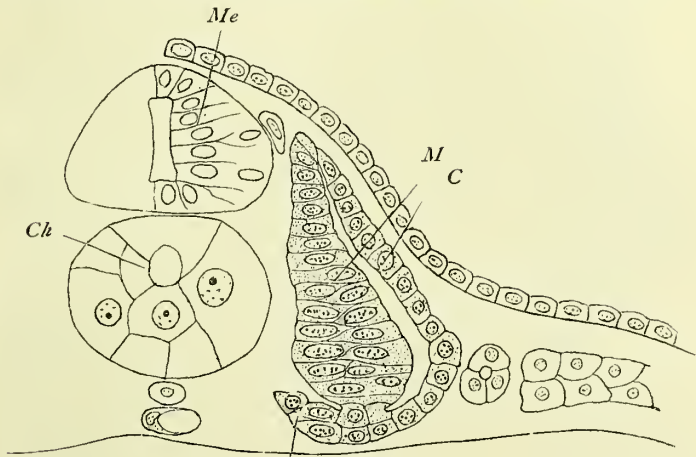
S Abb. 131.
