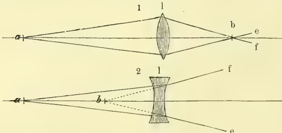
1 Gang der Lichtstrahlen durch eine Konverz., 2 durch eine Konkavlinse. a Leuchtender Objektspunkt — b Bildpunkt — l Linse — ef Richtung der Lichtstrahlen hinter dem Bildpunkte.
