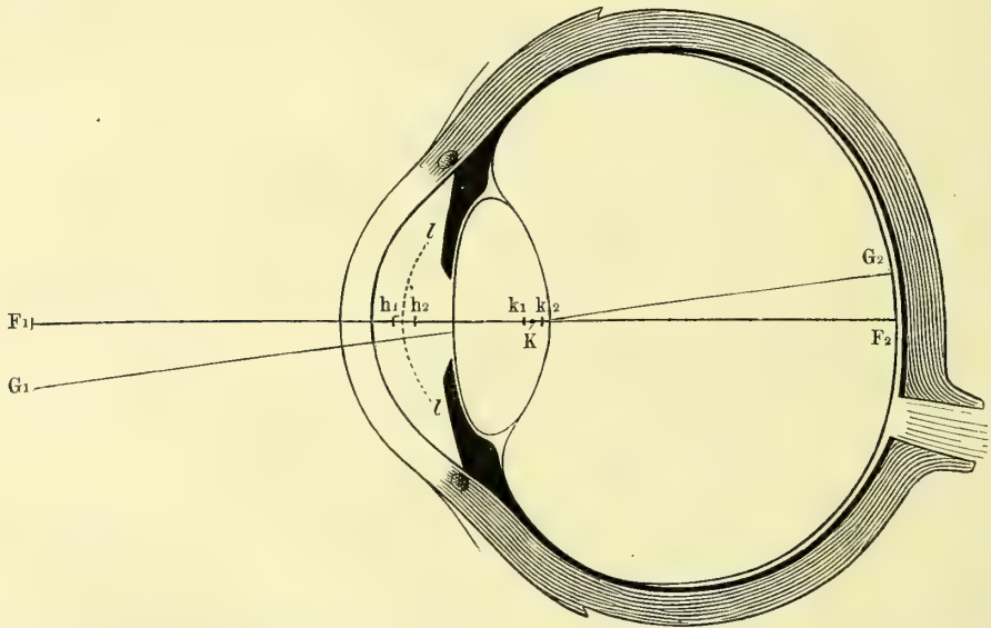
Schema des Ganges der Lichtstrahlen im Auge. F_1 F_2 Augennachse — G_1 G_2 Gesichtslinie — h_1 h_2 die Hauptpunkte, k_1 k_2 die Knotenpunkte des optischen Systemes des Auges. Im übrigen vgl. Text, S. 581.
