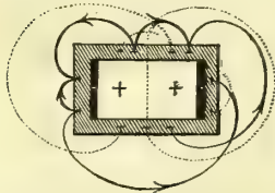
Schema der elektrischen Wirkung eines Muskel- oder Nervenstückes. Die Pfeile geben die Stromrichtung an, die punktierten Bögen bezeichnen die unwirksame Anordnung.
