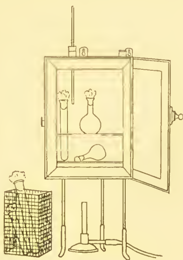
FIG. 2.—Hot-air steriliser.
