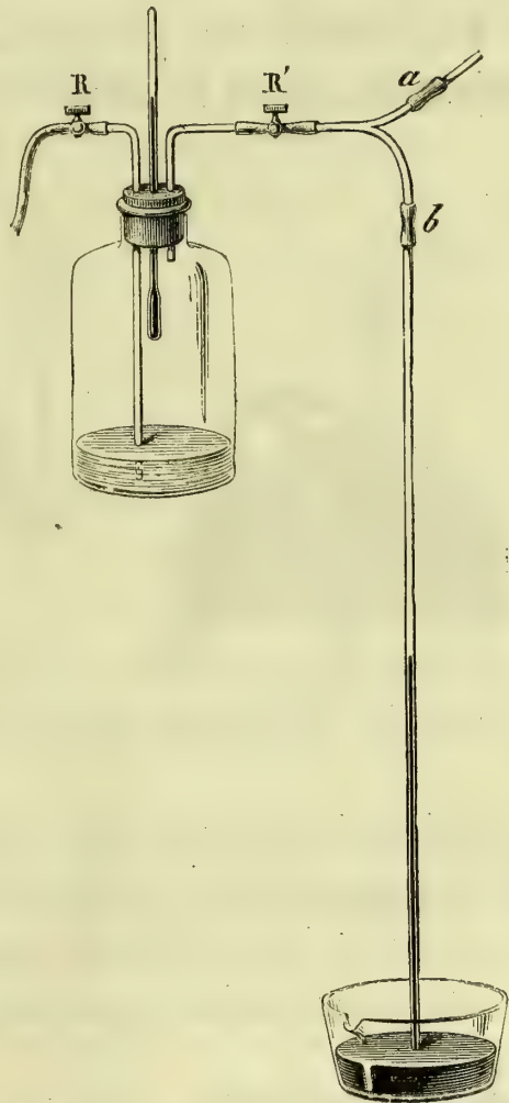
Fig. 41. — Flacon disposé pour la saturation du sang par l'oxygène sous diverses dépressions.
