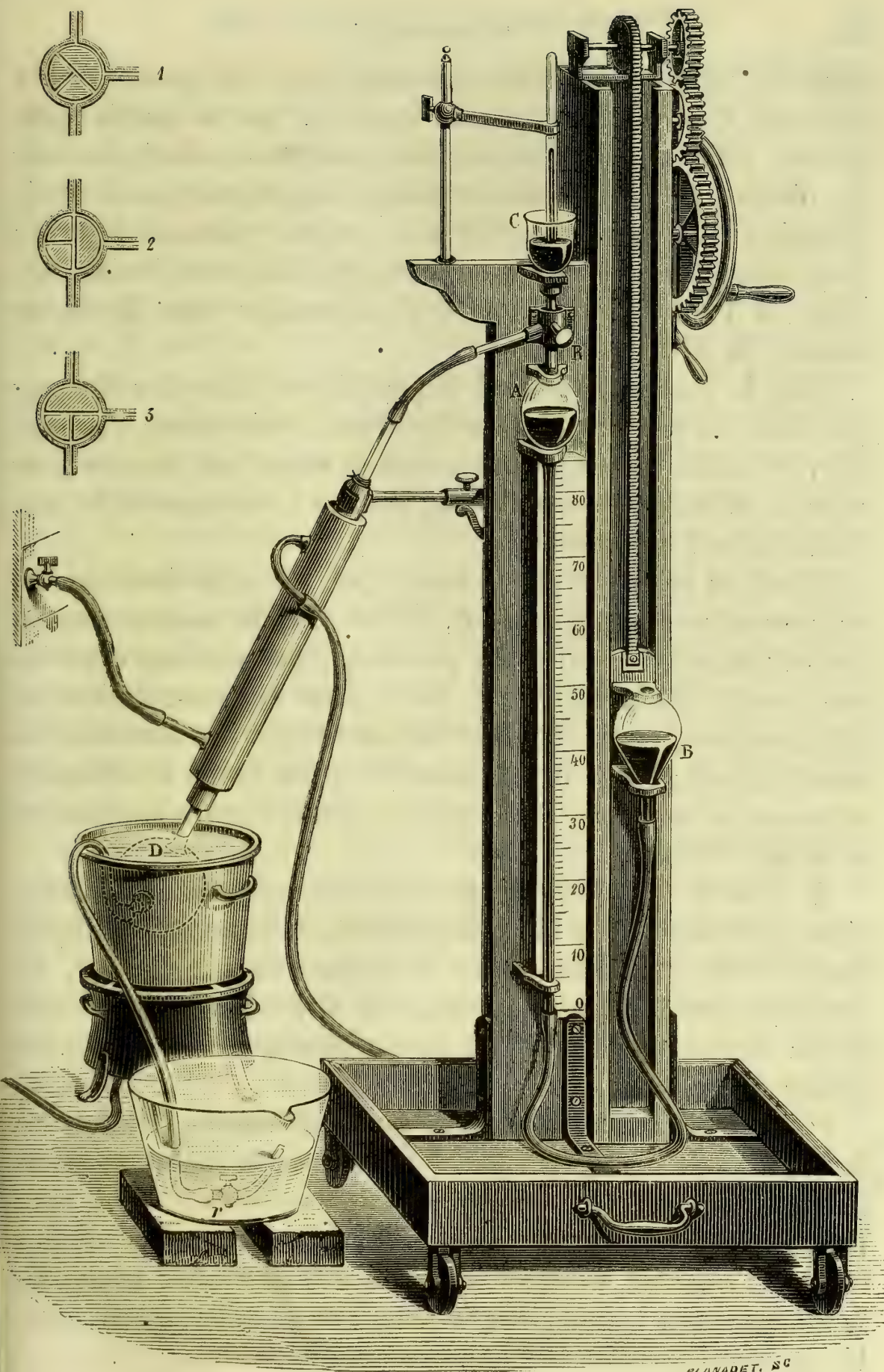
Fig. 16. — Pompe à mercure disposée pour l'extraction des gaz du sang.
