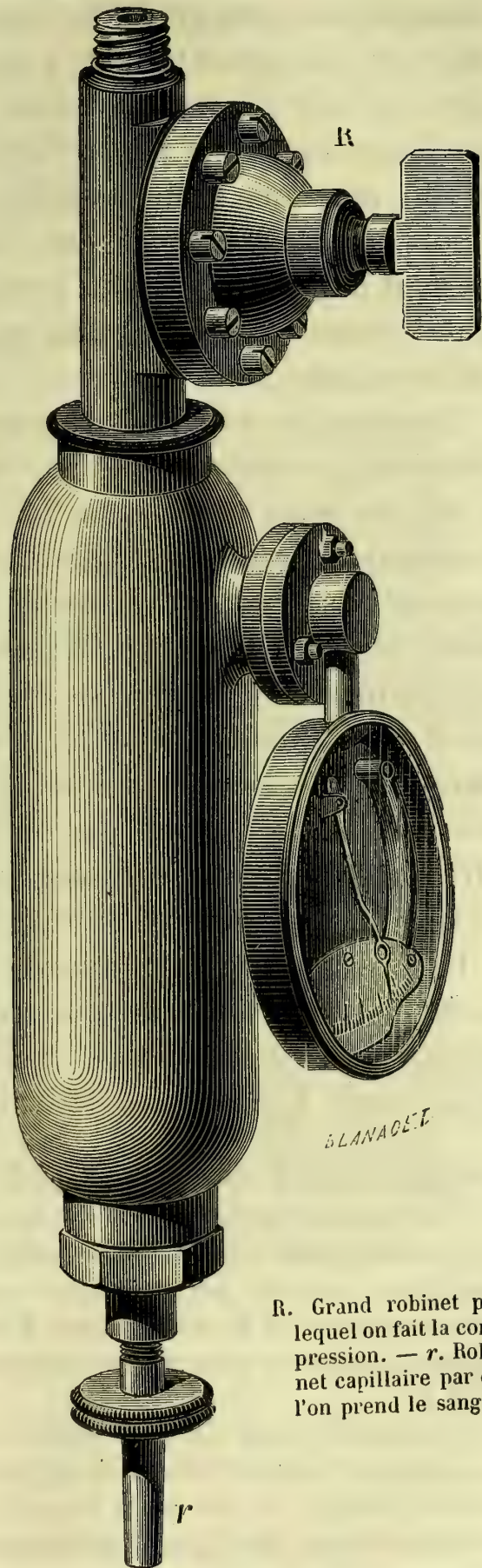
Fig. 45. — Appareil pour saturer d'air le sang à de hautes pressions.
