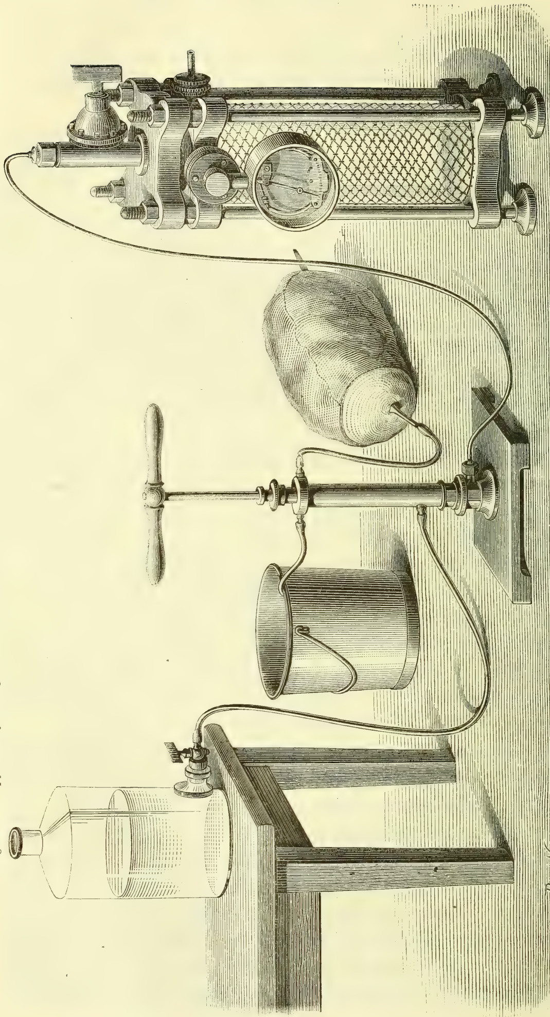
Fig. 20. — Appareil cylindrique en verre pour hautes pressions (25 atmosphères), en charge d'air suroxygéné.
