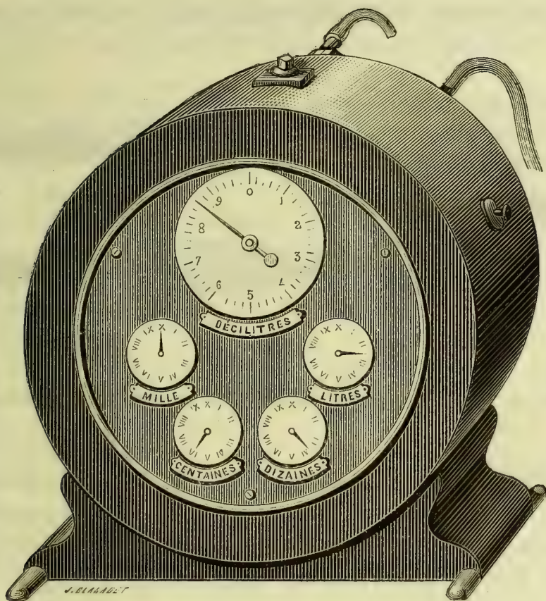
Fig. 65. — Compteur à gaz pour la mesure des mouvements respiratoires.
