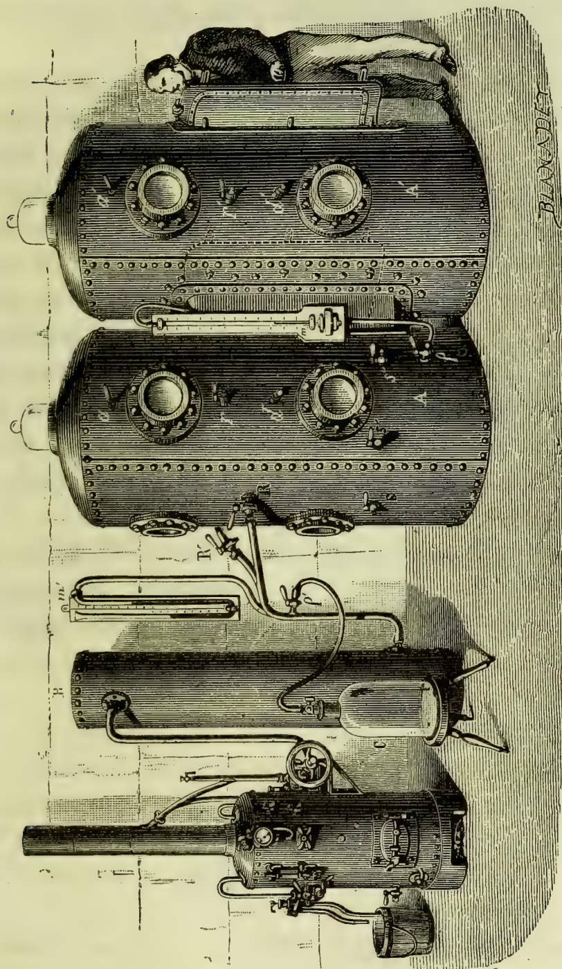
Fig. 27. — Grand appareil pour l'étude des faibles pressions.
