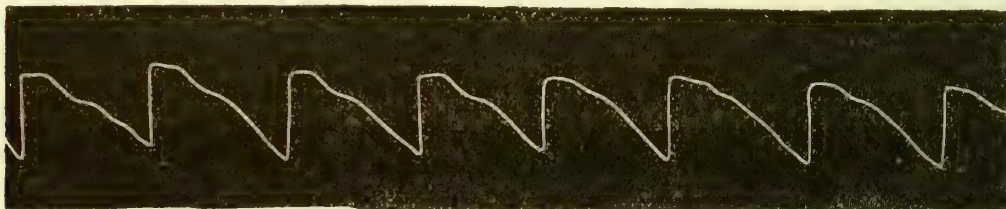
Fig. 85. — Pouls à Morges (580 m ), repos absolu (10 juillet).
