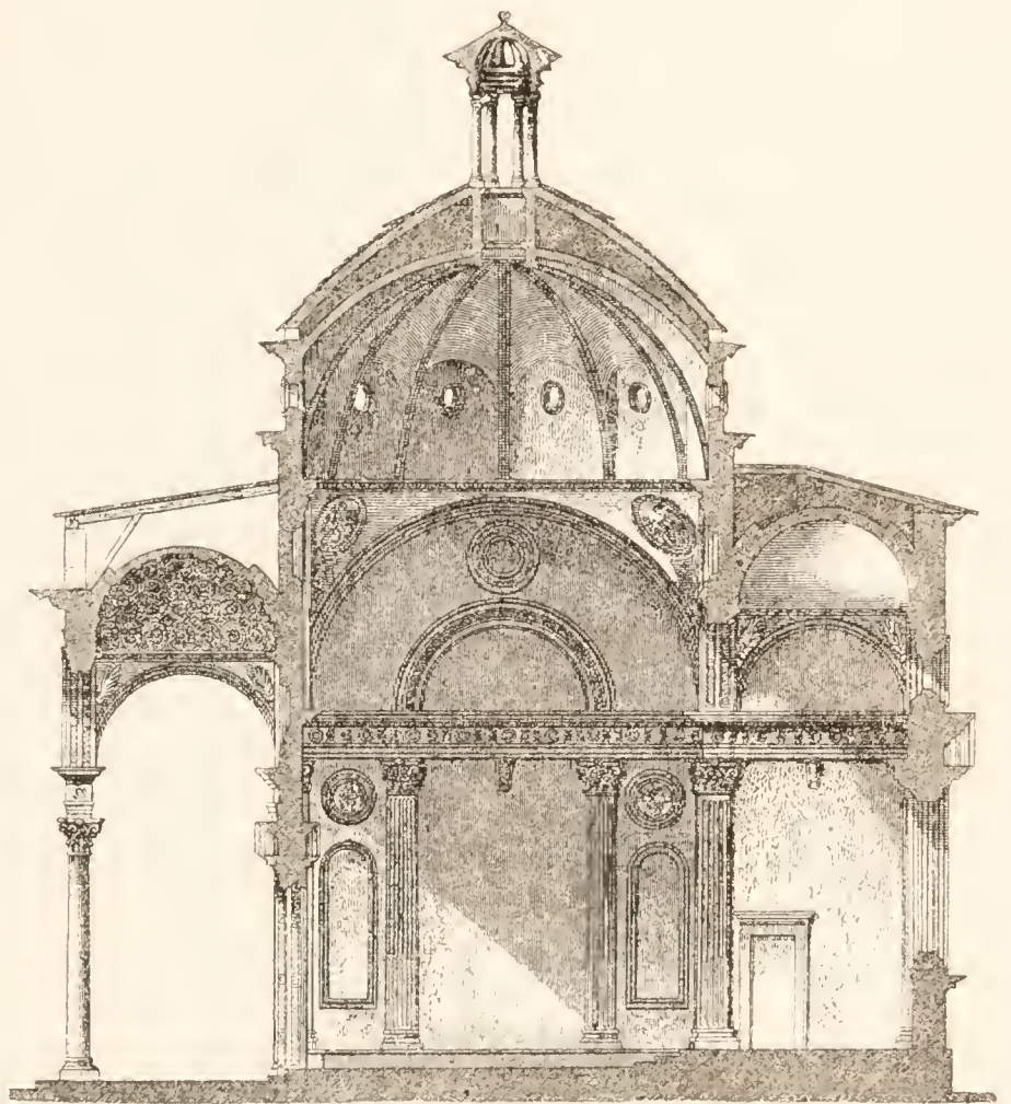
Fig. 69. Capp. Pazzi zu Florenz. Querschnitt. (Nach Paulus.)
