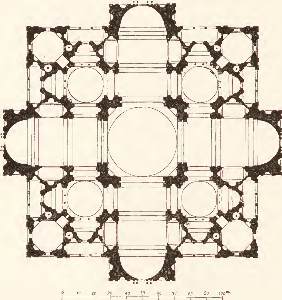
Fig. 83. St. Peter. Bramante's erster Grundriss.
