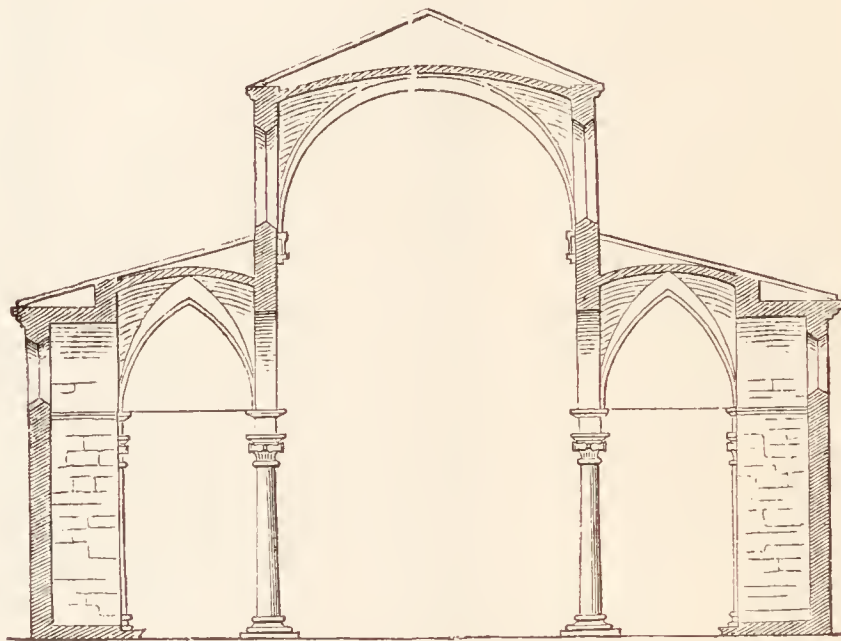
Fig. 117. Servi zu Siena. Querschnitt. (L.)
