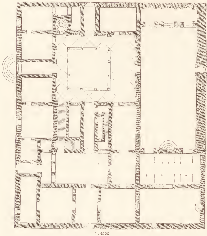
Fig. 159. Pal. Riccardi zu Florenz. Grundriss.
