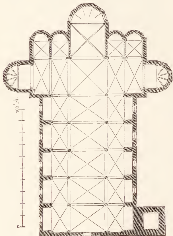
Fig. 116. Servi zu Siena. Grundriss. (L.)
