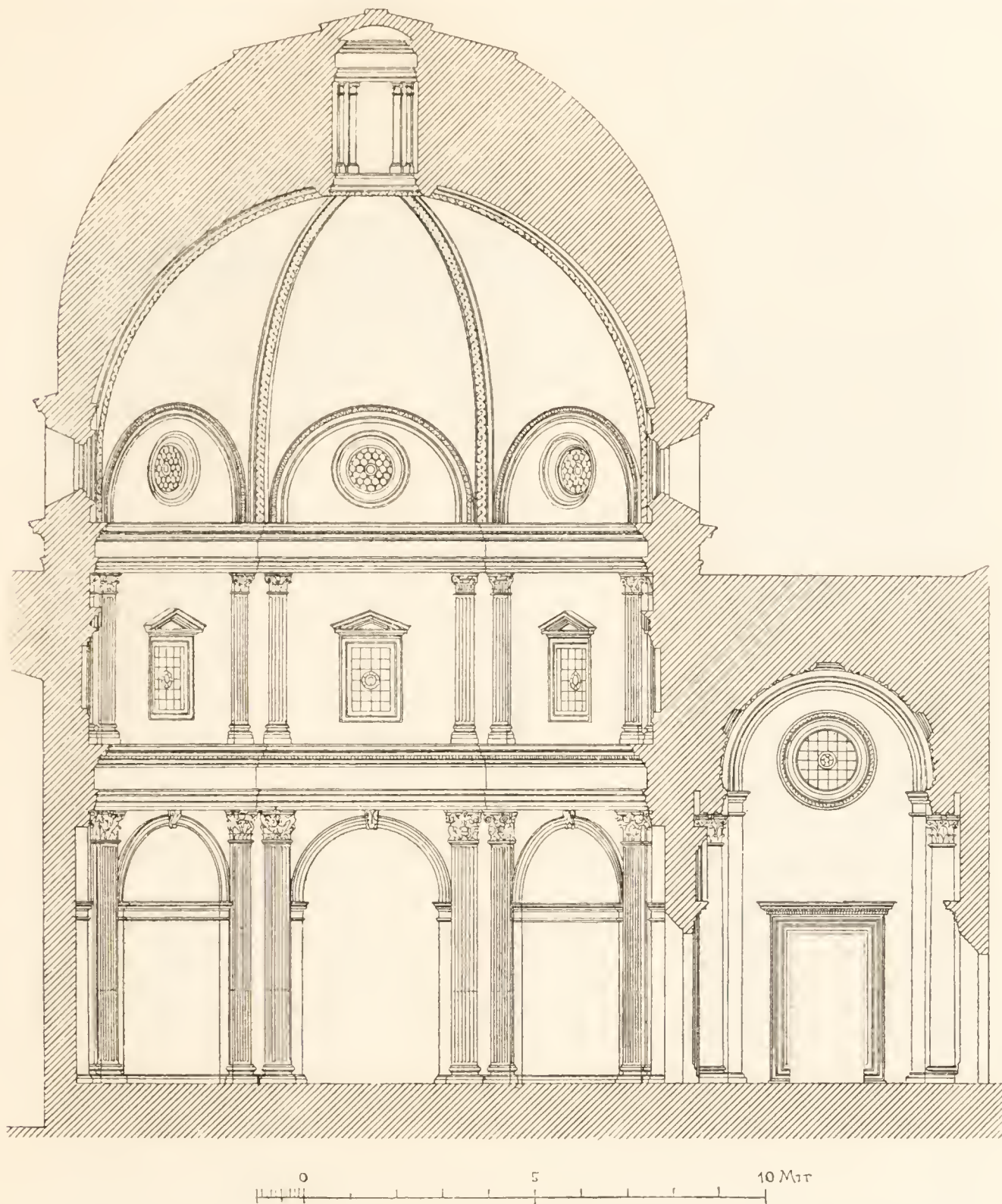
Fig. 144. Sacristei von S. Spirito in Florenz. Durchschnitt. (Nach Mayreder.)
