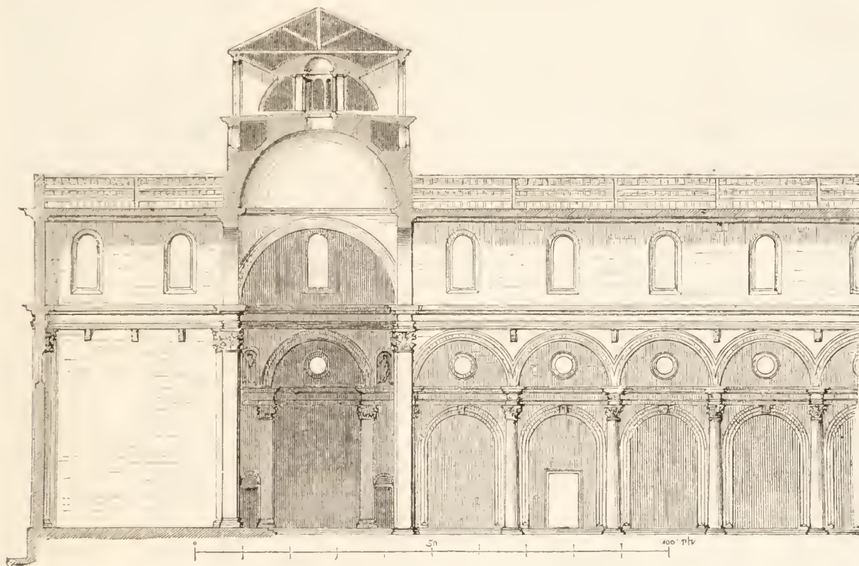
Fig. 113. S. Lorenzo zu Florenz. Längenschnitt.
