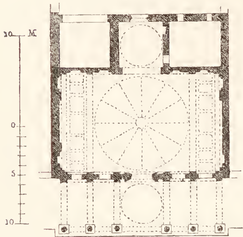
Fig. 67. Capp. Pazzi zu Florenz. Grundriss. (Nach Paulus.)
