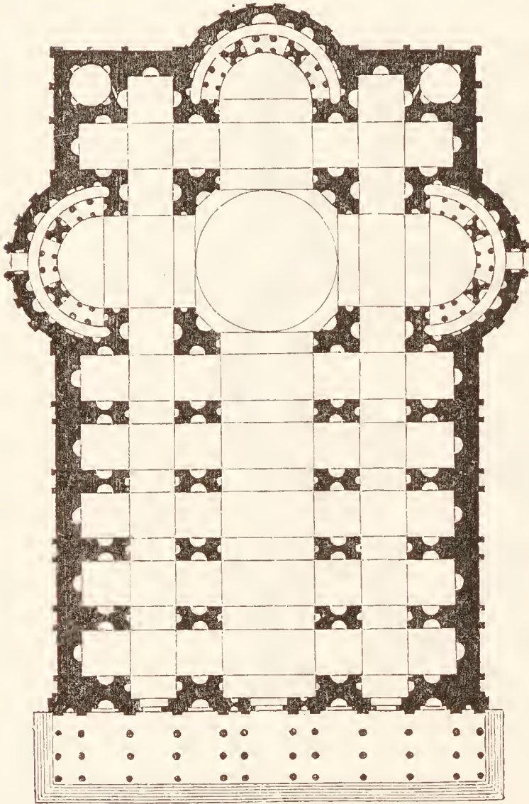
Fig. 85. St. Peter. Rafaels Grundriss. (Nach Serlios entstellter Reproduction.)
