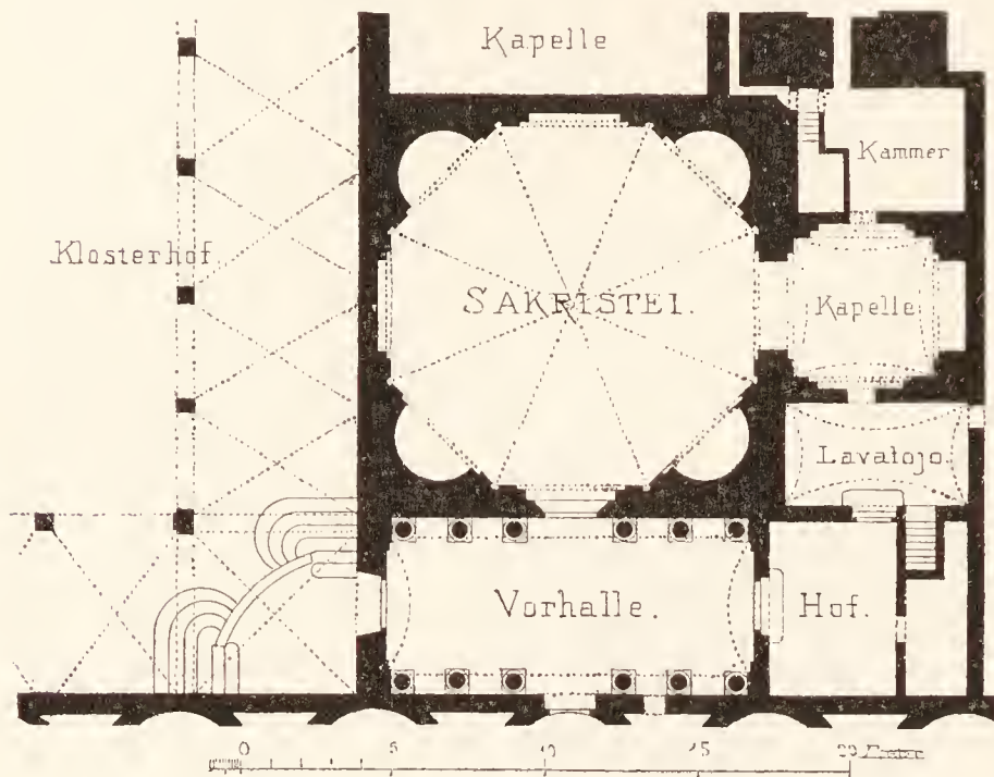
Fig. 143. Sacristei von S. Spirito in Florenz. Grundriss. (Nach Mayreder.)
