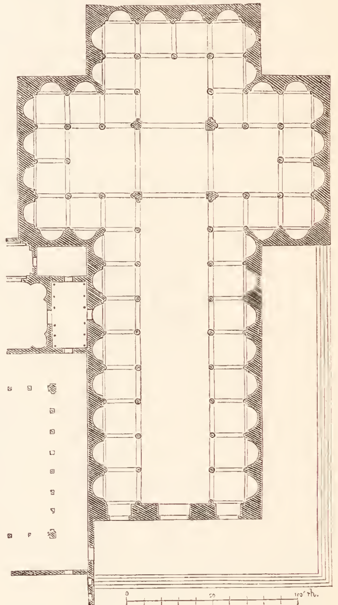
Fig. 112. S. Spirito zu Florenz. Grundriss.
