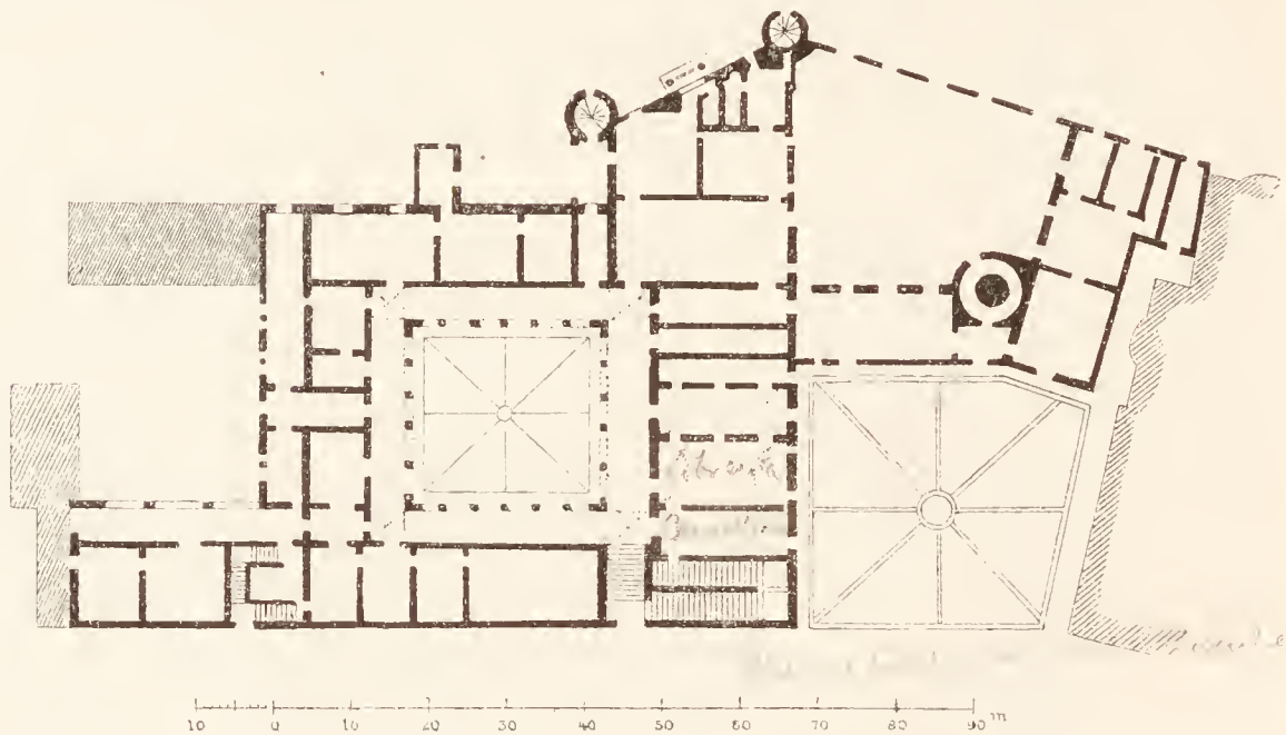
Fig. 164. Palast von Urbino. Grundriss.
