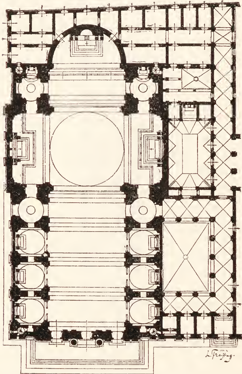
Fig. 126. Il Gesù in Rom. (Nach Gurlitt.)
