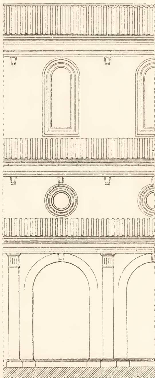
Fig. 149. S. Lorenzo in Florenz. Theilaufriss der Langseiten. (Nach Bühlmann.)
