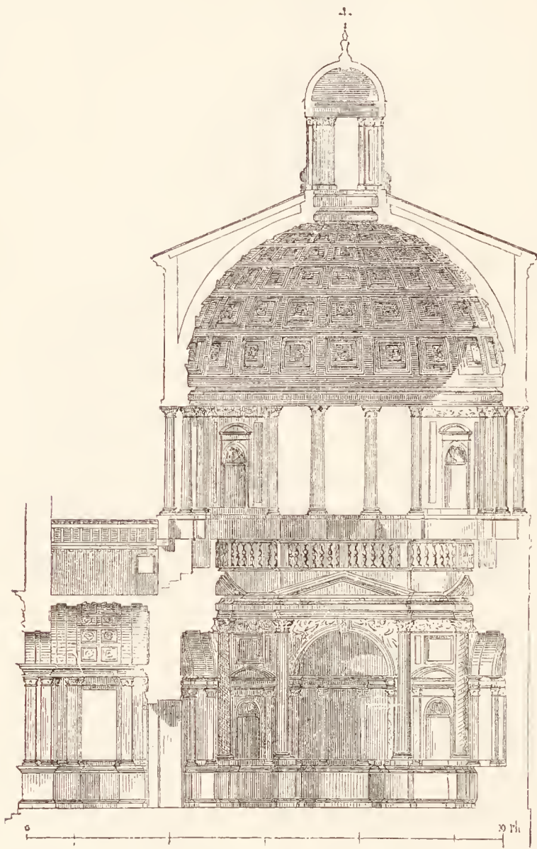
Fig. 92. Capp. Pellegrini in S. Bernardino zu Verona.
